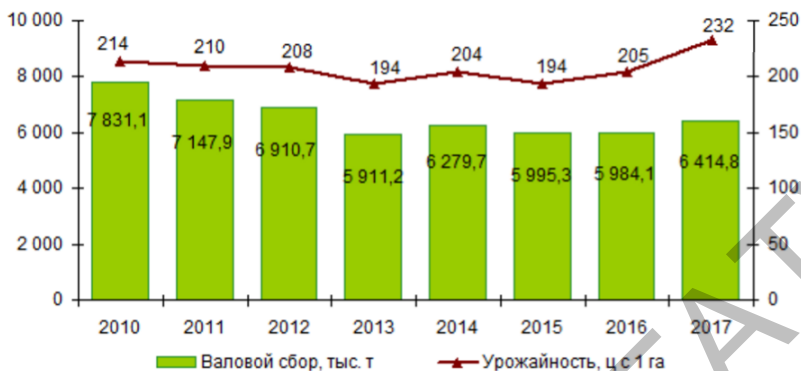
Рисунок – Динамика валового сбора и урожайности картофеля в хозяйствах всех категорий
