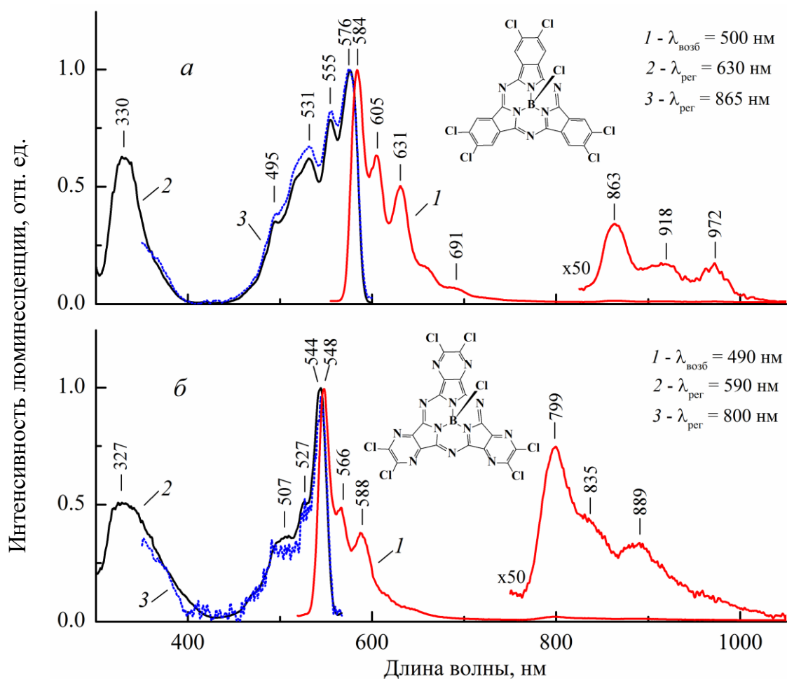
Спектры люминесценции (1), возбуждения флуоресценции (2) и возбуждения фосфоресценции (3) 1 (а) и 2 (б) в смеси растворителей толуол–диэтиловый эфир–йодистый метил при 77 °К. На вставках структурные формулы 1 и 2
