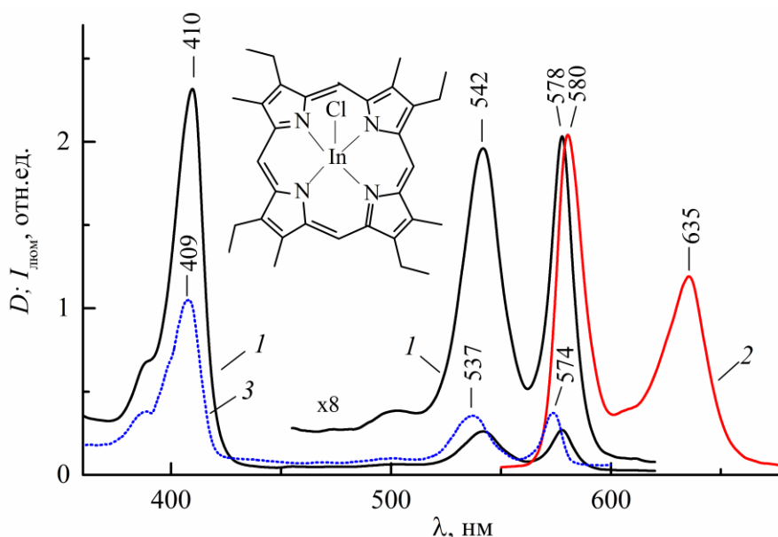
Рис. 1. Спектры поглощения (1), флуоресценции (2) при \lambda_{\text{возб}} = 409 нм InCl-EtioP-I в толуоле при 298 К и спектр возбуждения фосфоресценции (3) при \lambda_{\text{рег}} = 709 нм InCl-EtioP-I в смеси толуол:диэтиловый эфир (1:2) при 77 К. На вставке структурная формула InCl-EtioP-I
