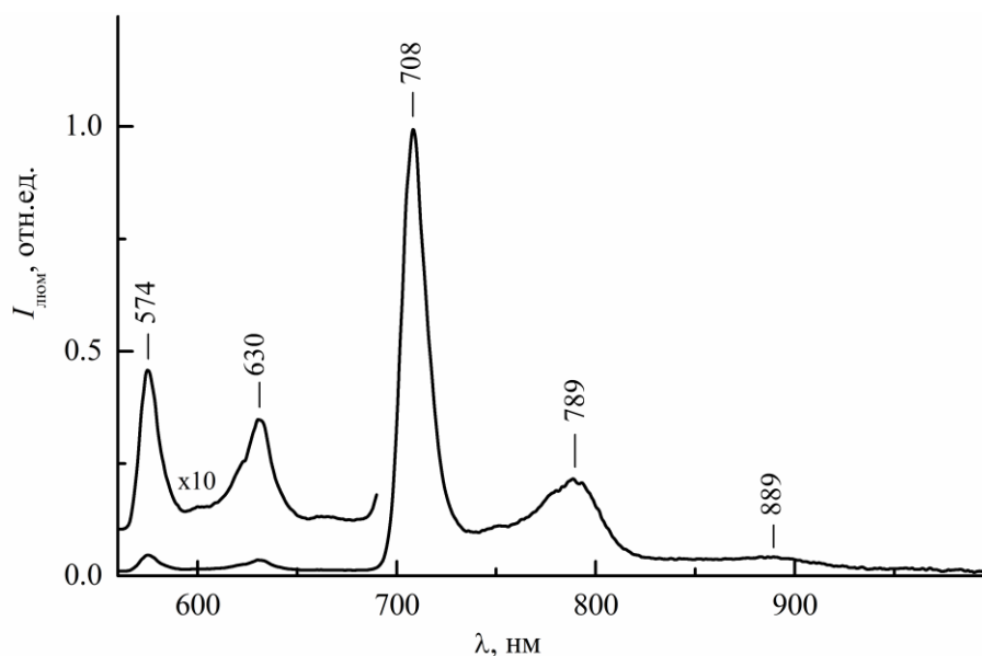
Рис. 2. Спектр люминесценции при \lambda_{\text{возб}} = 409 нм InCl-EtioP-I в смеси толуол:диэтиловый эфир (1:2) при 77 К.
