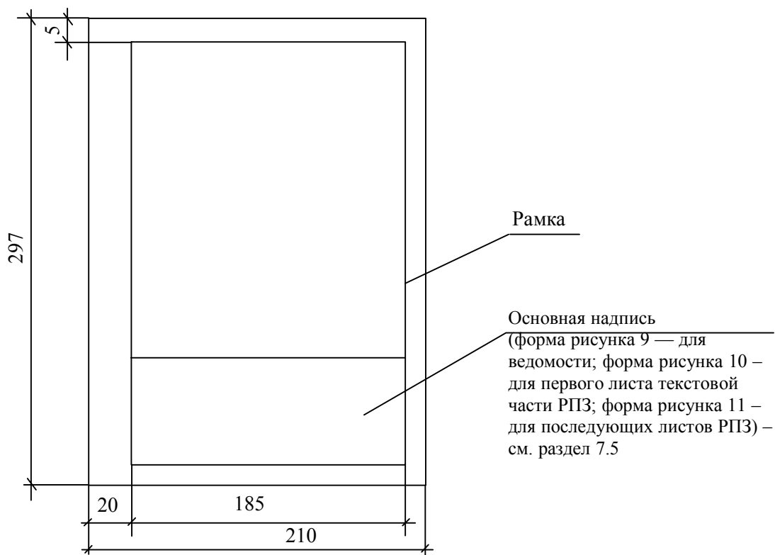
Рисунок 1 – Компонировка и размеры листа текстовой части РПЗ
