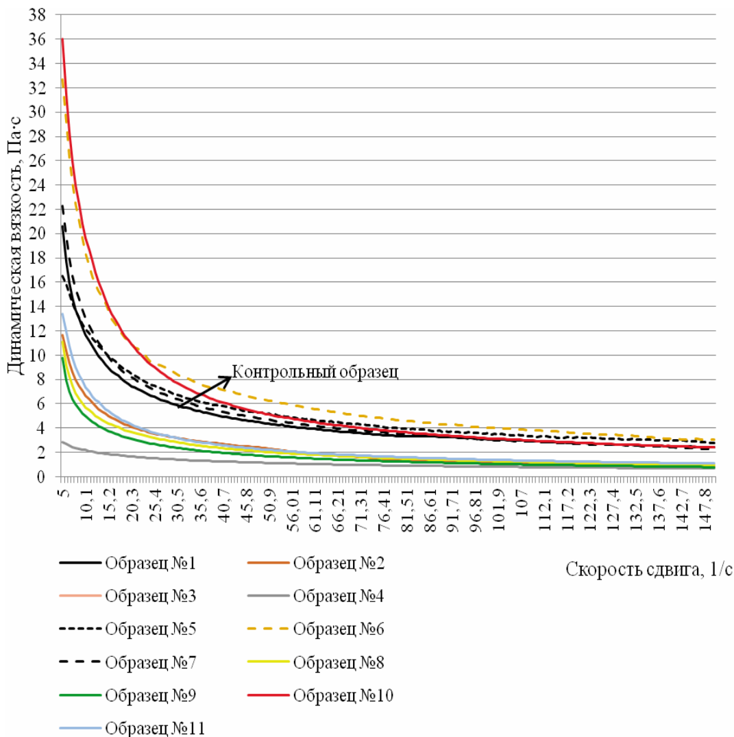
Рис. 2. Изменение динамической вязкости лабораторных образцов низкобелкового картофельного пюре в зависимости от скорости сдвига Fig. 2. Change in dynamic viscosity of laboratory samples of low-protein mashed potatoes depending on the shear rate
