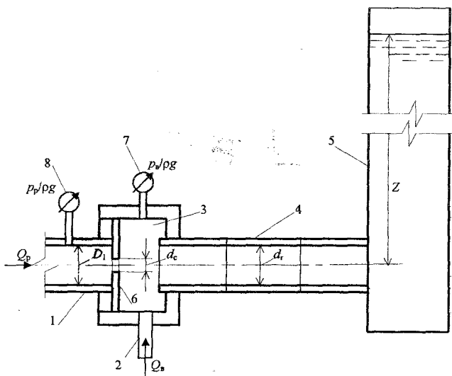
Рис. 1. Схема эжектора с переменной длиной горловины и соплом в виде диафрагмы с прямоугольными кромками: 1 — подводящая труба; 2 — воздушная трубка; 3 — воздушная камера (камера смешения); 4 — горловина; 5 — прозрачная стеклянная труба; 6 — диафрагма с прямоугольными кромками; 7 — вакуумметр; 8 — манометр
