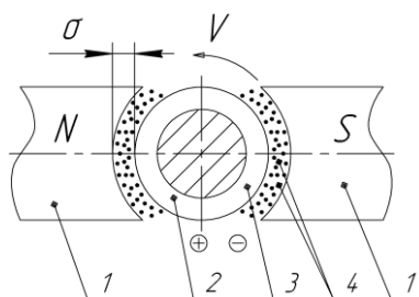
Рис. 2. Схема магнитно-абразивной обработки:
