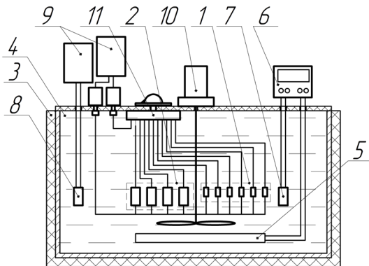
Рисунок 4 – Схема установки для изучения температурной зависимости сопротивления проводников и полупроводниковых приборов
