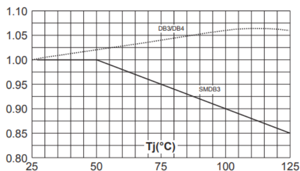
Рисунок 2 – Относительное падение электропроводности динистора SMDB3 производства STMicroelectronics (PФ)
