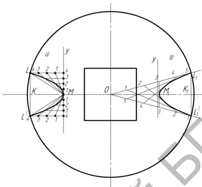
Рисунок 2 - Варианты параболического профиля желобка высевальной катушки
