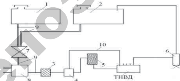
Рисунок 2. Схема системы питания трактора «БЕЛАРУС-80.1» для работы на биотопливе: 1, 2 – топливные баки; 3 – фильтр грубой очистки; 4 – топливоподкачивающий насос; 5 – фильтр тонкой очистки; 6 – форсунка; 7 – трехходовой кран; 8 – подогреватель воздуха; 9, 10 – топливopроводы
