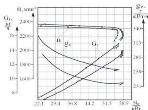
Рисунок 1. Регуляторные характеристики дизеля Д-243 при работе:
