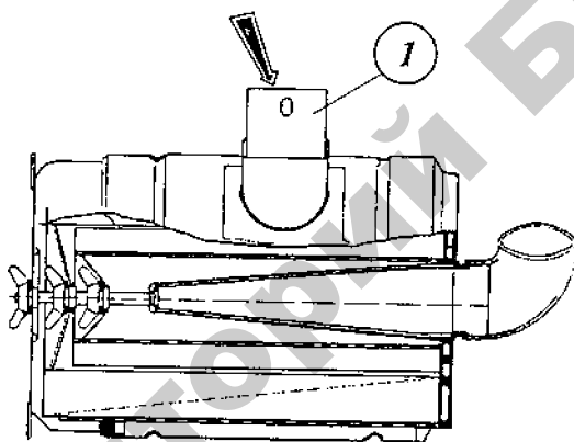
Рис. 3.19. Проверка герметичности соединений воздухоочистителя и впускного тракта:
