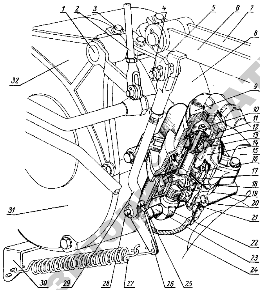
Рис. 3.43. Тормозной кран и его привод (МТЗ-80):
