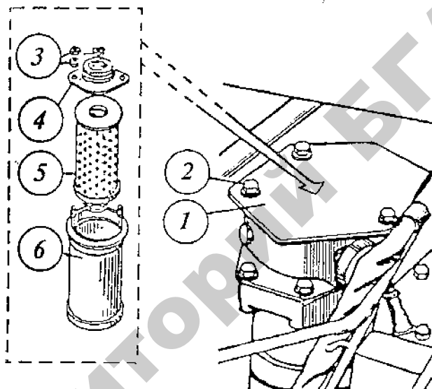
Рис. 3.34. Схема замены фильтрующего элемента гидросистемы трактора «Беларус-1221»:
