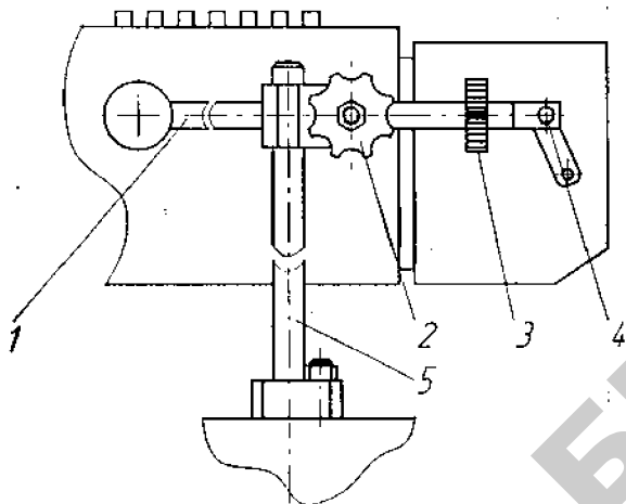
Рис. 2.21. Устройство натяжное:
