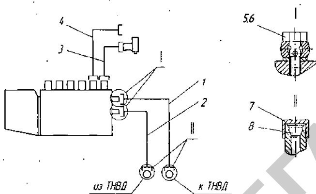
Рис. 2.15. Схема соединений трубопроводов при испытании 4ТМ 8,5×10
