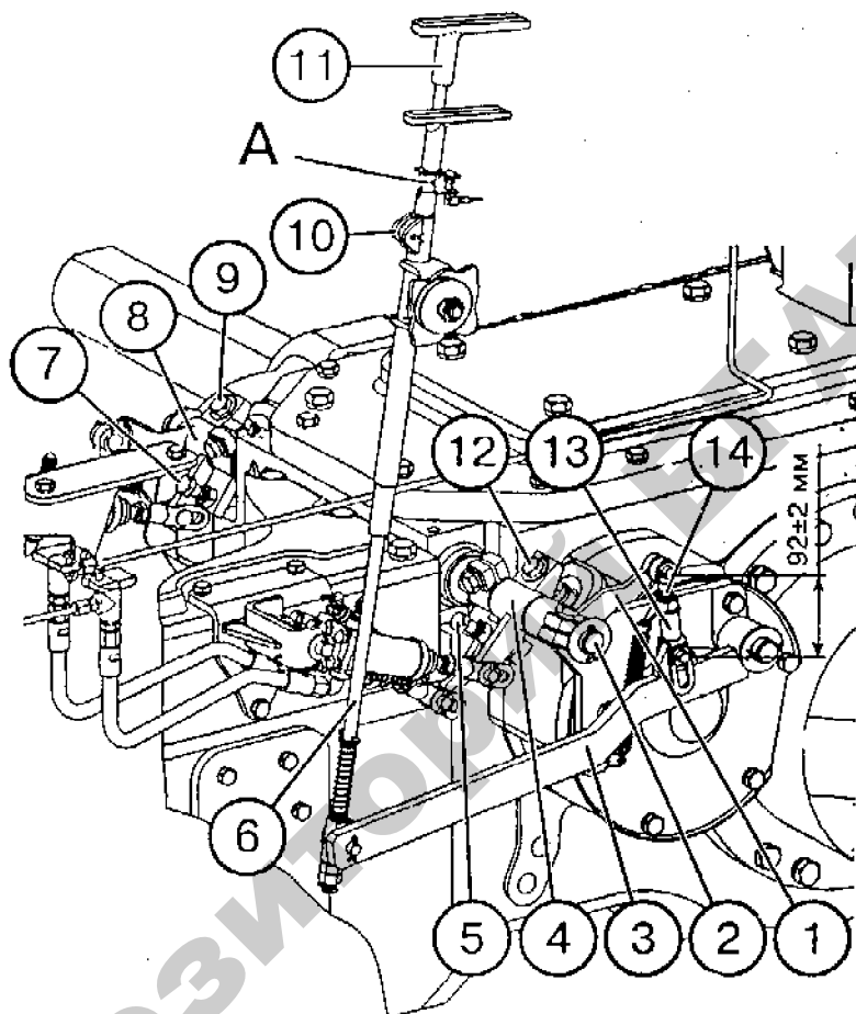
Рис. 3.33. Схема регулировки стояночного тормоза:
