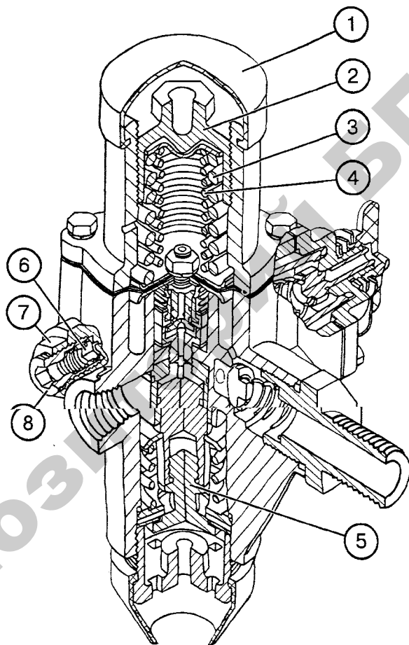
Рис. 3.42. Регулятор давления трактора «Беларус-1522»:
