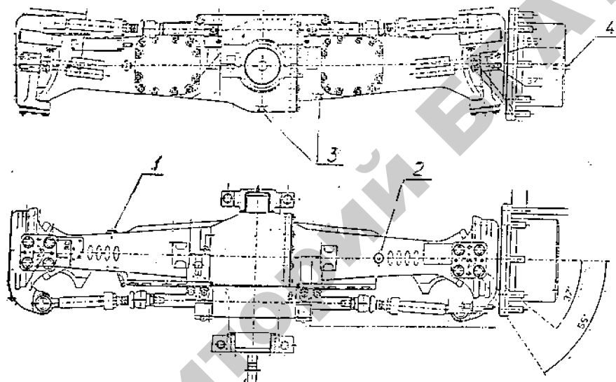
Рис. 3.23. Схема замены масла в картере ПВМ трактора «Беларус-2522»: 1, 2, 3, 4 – пробки
