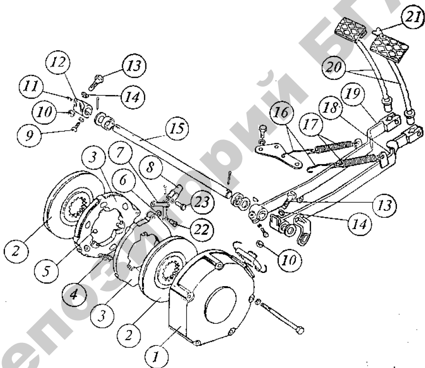
Рис. 3.29. Рабочий тормоз и управление трактора «Беларус-1221»:
