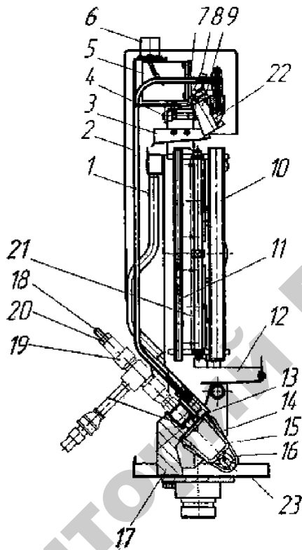
Рис. 2.7. Блок мерный:
