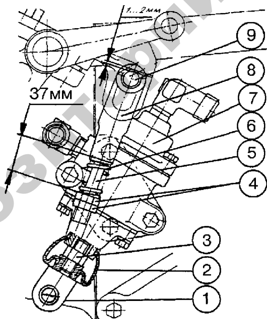
Рис. 3.44. Регулировка тормозного крана трактора «Беларус-1221»:
