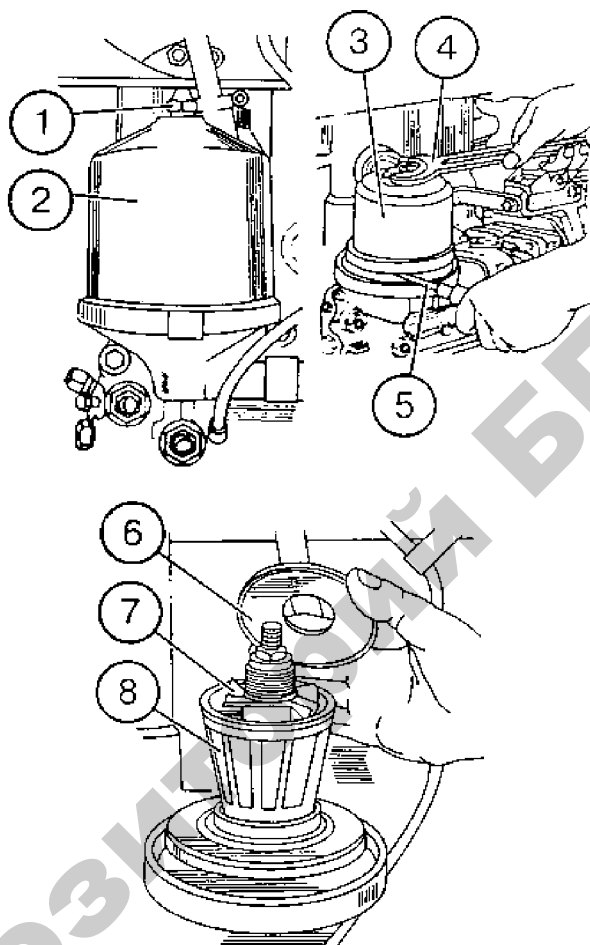
Рис. 3.13. Очистка ротора центробежного масляного фильтра дизеля:
