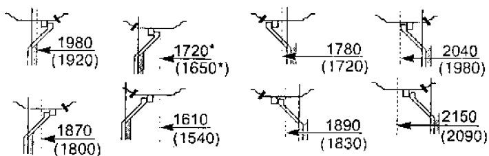
Рис. 3.60. Схема установки колеи по передним колесам тракторов «Беларус-1522, -1523»
