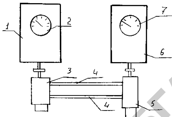
Рис. 3.69. Принципиальная схема установки для послеремонтной обкатки аксиально-плунжерных гидронасосов и гидромоторов:
