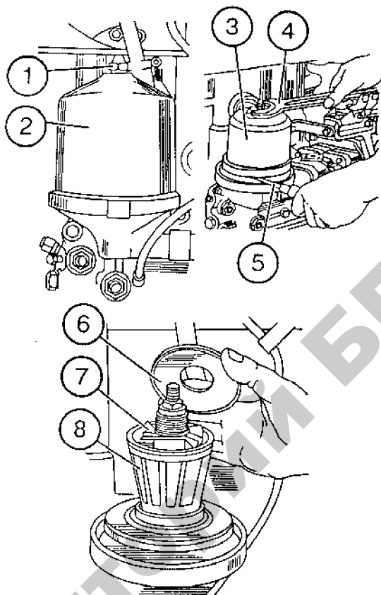
Рис. 3.20. Схема очистки роторов центробежного масляного фильтра КПП трактора «Беларус-2522, -1522»: 1 – гайка; 2 – колпак; 3 – ротор; 4 – ключ гаечный; 5 – отвертка; 6 – крышка; 7 – крыльчатка; 8 – фильтр сетчатый
