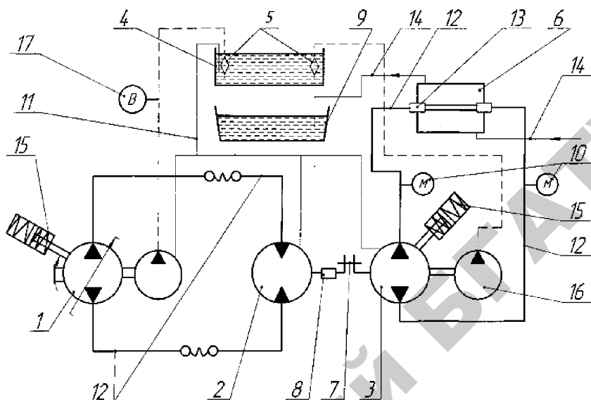
Рис. 3.71. Гидравлическая схема обкаточно-диагностического стенда:
