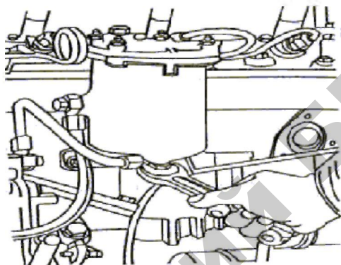
Рис. 3.51. Слив отстоя из фильтра тонкой очистки топлива
