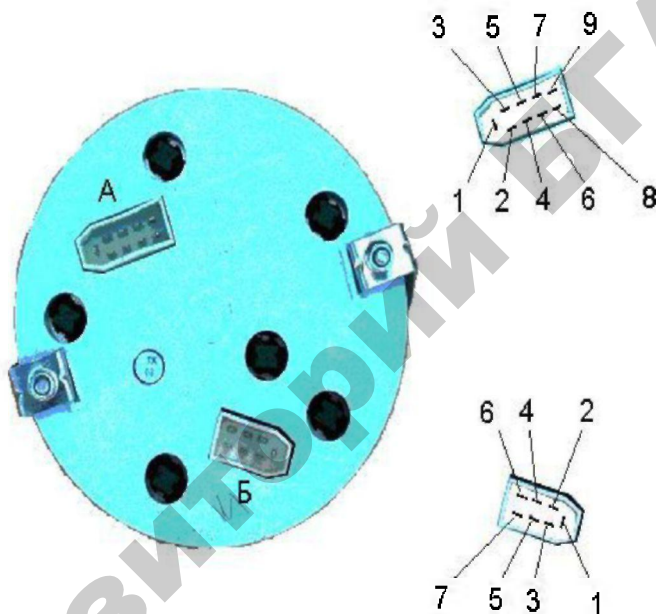
Рис. 2.55. Общий вид задней стенки комбинированного прибора и цоколевка проводов:
