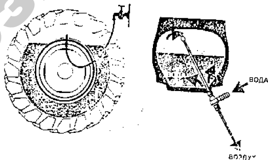
Рис. 3.68. Балластирование колес заполнением шин жидкостью
