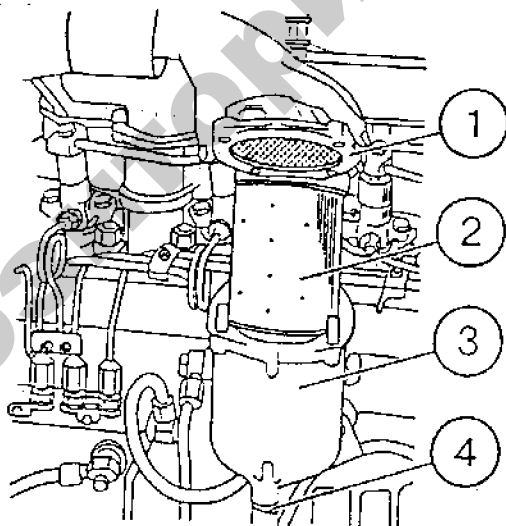
Рис. 3.15. Замена фильтрующего элемента фильтра тонкой очистки топлива трактора «Беларус-2522»:
