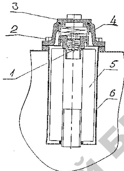
Рис. 3.36. Схема замены фильтрующего элемента гидросистемы трактора «Беларус-2522»:
