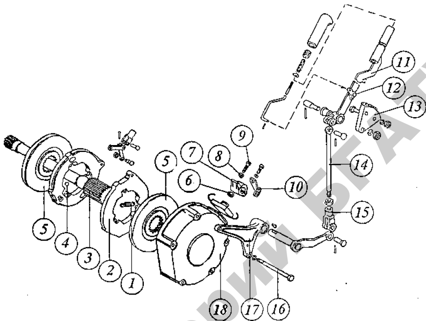
Рис. 3.30. Стояночно-запасной тормоз и управление трактора «Беларус-1221»:
