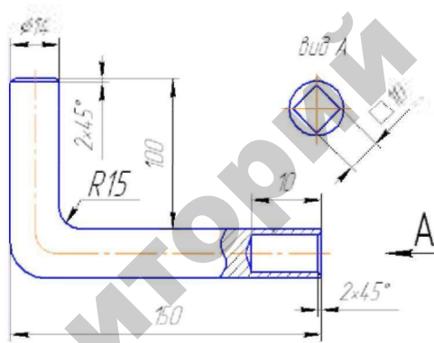
Рис. 3.5. Ключ для выворачивания гнезда предохранительного клапана
