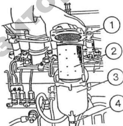
Рис. 3.52. Замена фильтрующего элемента: 1 – крышка; 2 – фильтрующий элемент; 3 – корпус; 4 – пробка
