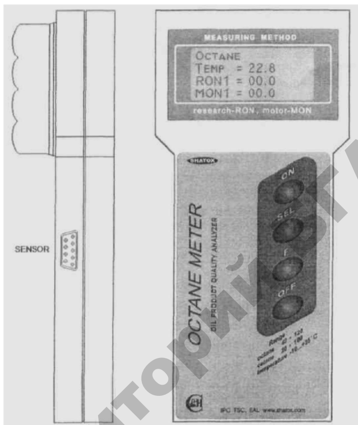
Рис. 3.76. Внешний вид октанометра (электронный блок)
