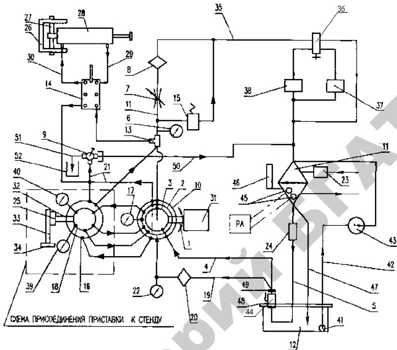
Рис. 2.3. Схема стенда гидромеханическая:
