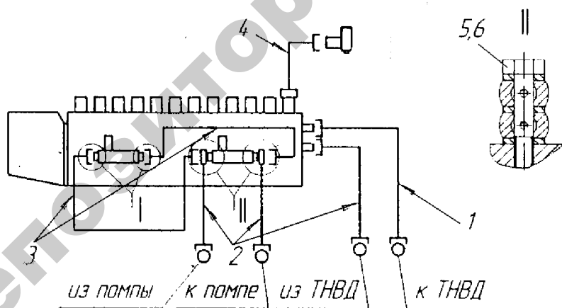
Рис. 2.20. Схема соединения топливопроводов при испытании ТНВД двигателя ЯМЗ-740 со шгатым топливоподкачивающим насосом:
