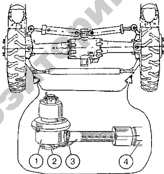
Рис. 3.28. Схема проверки люфта рулевого управления: 1 – шарнир рулевой тяги; 2 – резьбовая пробка; 3 – проволока; 4 – рулевая тяга
