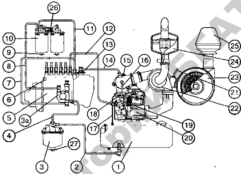
Рис. 3.47. Схема системы питания.
