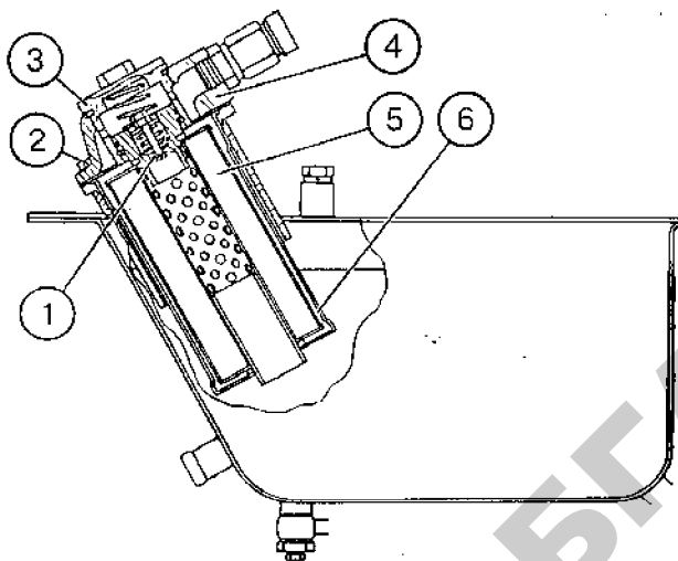
Рис. 3.35. Схема замены фильтрующего элемента гидросистемы трактора «Беларус-1522»:
