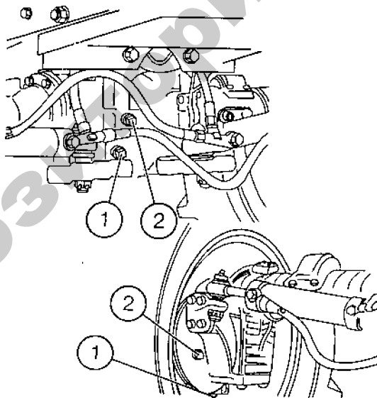
Рис. 3.22. Схема замены масла в главной передаче и колесных редукторах ПВМ трактора «Беларус-1522»:
