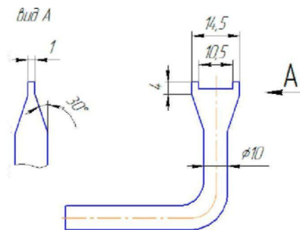
Рис. 3.4. Специальная отвертка для разборки и сборки клапанов бустера
