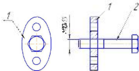
Рис. 3.2. Устройство подпора перепускного клапана распределителя: 1 – крышка перепускного клапана; 2 – болт
