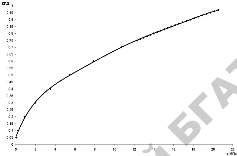
Рис. 3.72. График зависимости объемного КПД насоса от его давления при диаметре дросселя 6,2 мм
