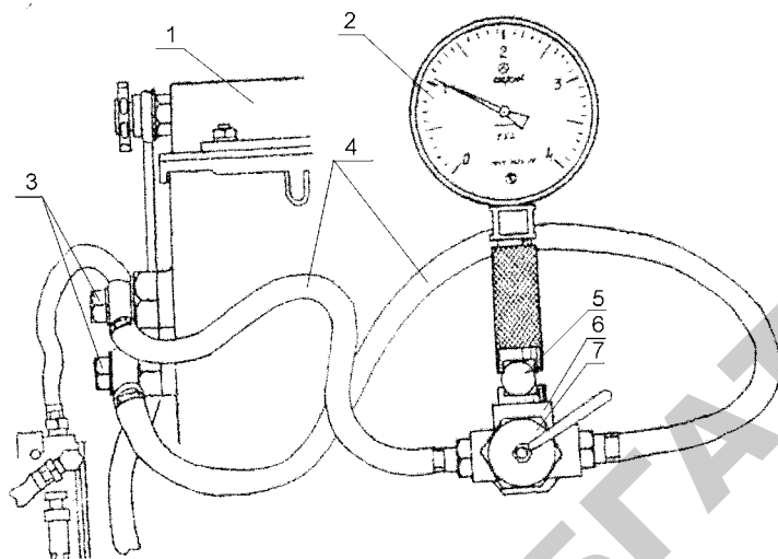
Рис. 3.50. Диагностирование с помощью устройства КИ-4801-ГОСНИТИ фильтра тонкой очистки топлива, перепускного клапана и подкачивающего насоса: 1 – фильтр тонкой очистки топлива; 2 – манометр; 3 – удлиненные штуцера; 4 – шланги; 5 – клапан; 6 – корпус; 7 – 3-ходовой кран
