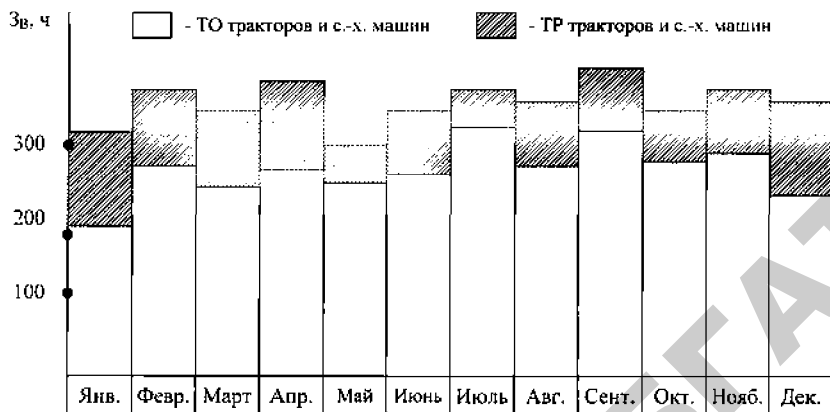
Рис. 4.3. График затрат рабочего времени специализированного звена
