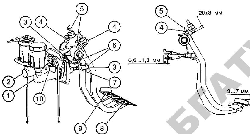
Рис. 3.31. Схема регулировки хода педалей: 1, 2 – гидроцилиндры; 3 – вилки; 4, 7 – контргайки; 5 – болты; 6 – пальцы; 8 – левая педаль тормоза; 9 – правая педаль тормоза
