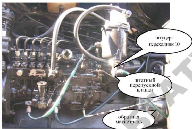
Рис. 2.51. Топливная система трактора МТЗ после установки ДРТ
