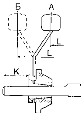
Рис. 3.61. Схема установки задних колес на ступицу тракторов «Беларус-1522, -1523» и измерения размера K
