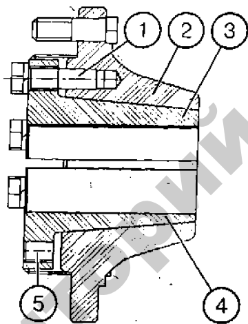
Рис. 3.59. Ступица ведущих задних колес тракторов «Беларус-1522, -1523»:
