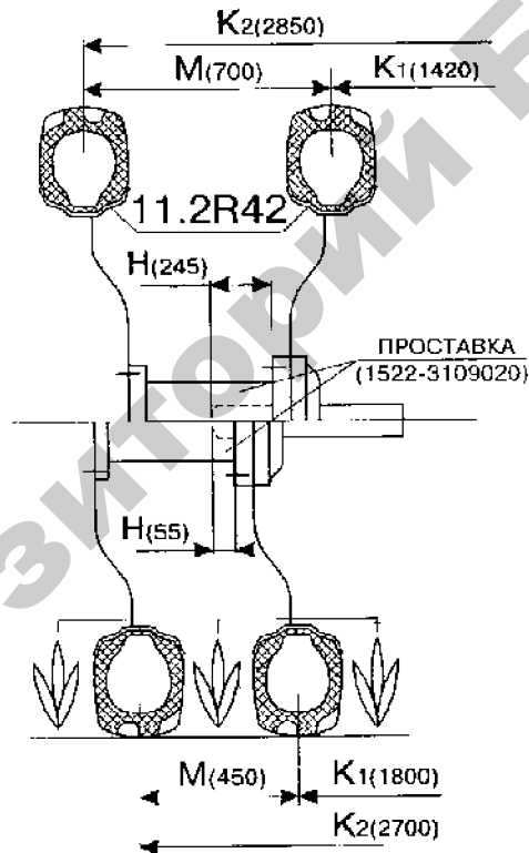
Рис. 3.64. Схема спаривания задних колес тракторов «Беларус-1522, -1523» для междурядной обработки пропашных культур на шинах дополнительной комплектации 11,2R28
