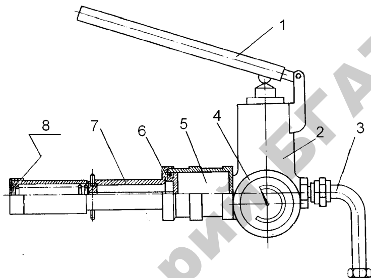
Рис. 3.48. Прибор КИ-9917-ГОСНИТИ для проверки форсунок: 1 – рычаг; 2 – корпус; 3 – топливопровод высокого давления; 4 – манометр; 5 – резервуар для топлива; 6 – поршень; 7 – ручка; 8 – пружина
