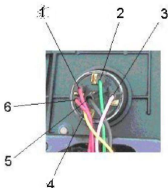
Рис. 2.53. Замок зажигания (вид сзади):
