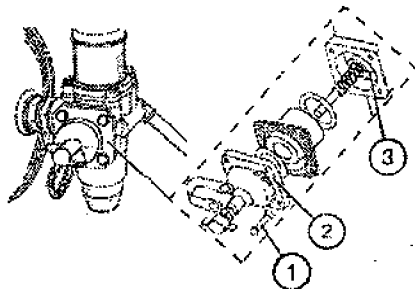
Рис. 3.37. Фильтрующий элемент регулятора давления пневмосистемы. 1 – болт; 2 – крышка; 3 – фильтрующий элемент
