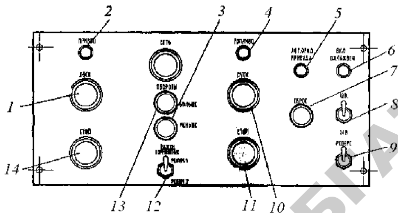
Рис. 2.10. Панель управления:
