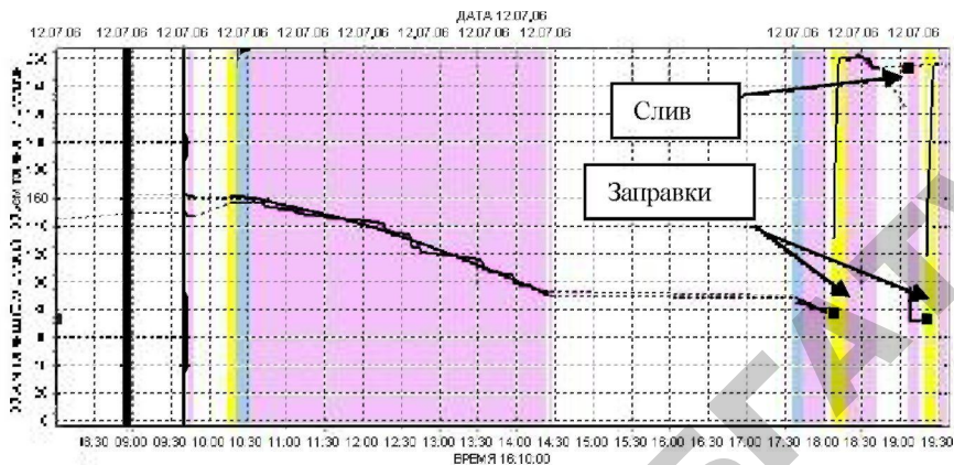
Рис. 2.63. Моменты слива и заправки
