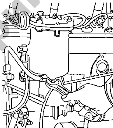
Рис. 3.18. Слив отстоя из фильтра тонкой очистки топлива дизеля трактора «Беларус-2522»
