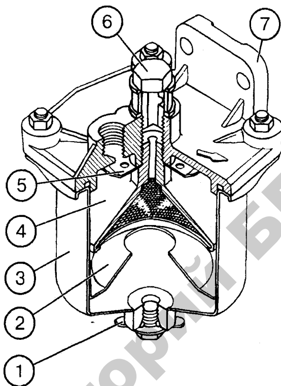
Рис. 3.49. Фильтр грубой очистки топлива:
