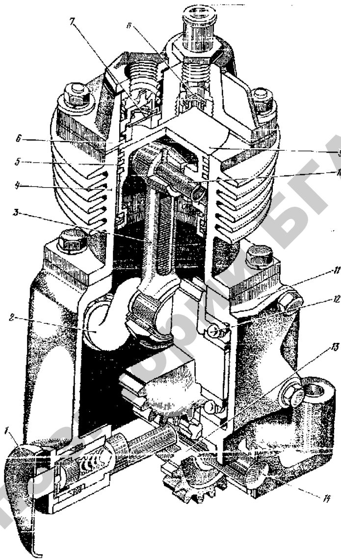
Рис. 3.45. Компрессор:
