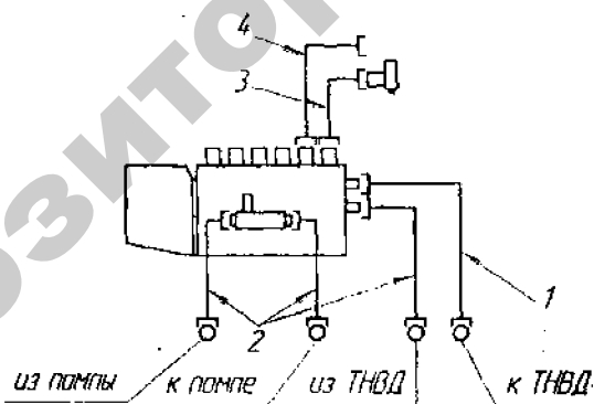
Рис. 2.16. Схема соединений топливопроводов при испытании ТНВД
