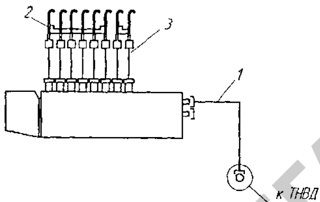
Рис. 2.19. Схема соединения топливопроводов при испытании ТНВД методом пролива:
