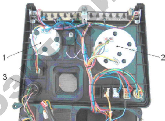
Рис. 2.52. Общий вид панели приборов с обратной стороны: 1 – тахоспидометр, 2 – комбинированный прибор, 3 – замок зажигания
