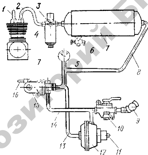
Рис. 3.38. Схема пневматической системы тракторов МТЗ-80/82:
