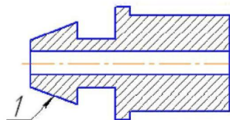
Рис. 3.6. Перепускной клапан: 1 – посадочное место перепускного (переливного) клапана
