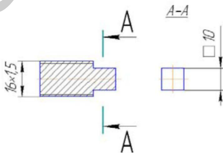
Рис. 3.1. Заглушка специальная предохранительного клапана
