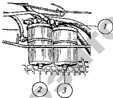
Рис. 3.17. Слив отстоя из фильтра тонкой очистки топлива дизеля тракторов «Беларус-1221, -1522»: 1, 2, 3 – пробки
