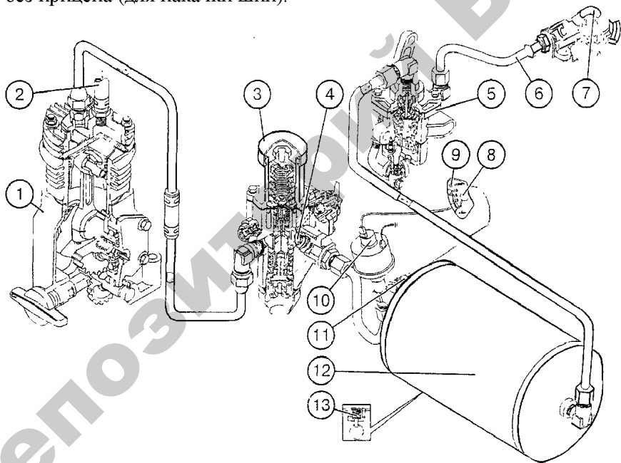
Рис. 3.39. Пневмопривод тормозов прицепа трактора «Беларус-1522»:
