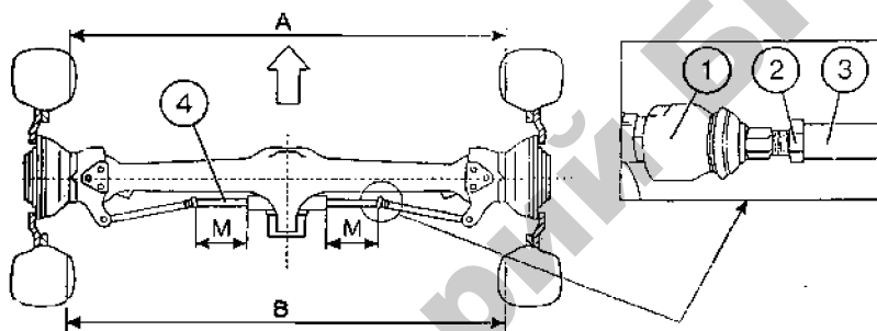
Рис. 3.26. Схема регулировки сходимости передних колес трактора «Беларус-1522»:
