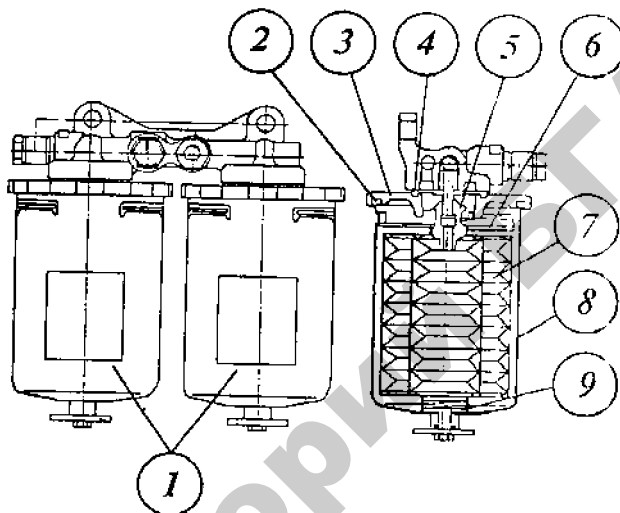
Рис. 3.16. Замена фильтрующих элементов тонкой очистки топлива дизелей тракторов «Беларус-1221, -1522»:
