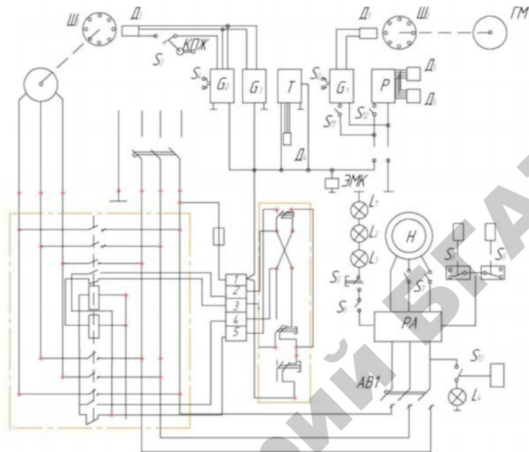
Рис. 2.4. Блок-схема электрическая.
