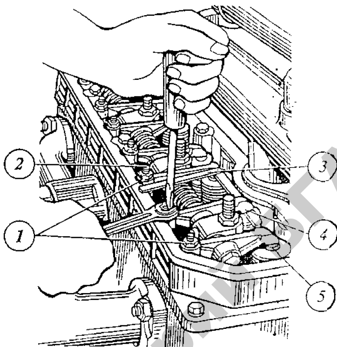
Рис. 3.11. Проверка и регулировка зазоров клапанов дизеля: 1 – контргайка; 2 – винт регулировочный; 3 – щуп; 4 – боек коромысла; 5 – стержень клапанов
