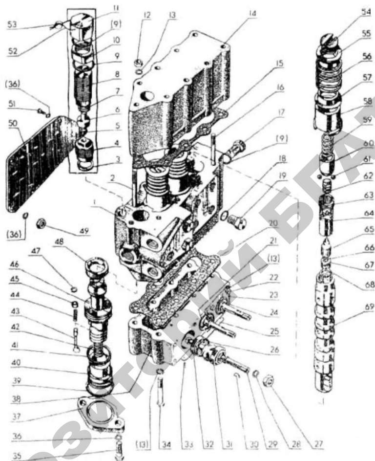
Рис. 3.10. Распределитель гидросистемы:
