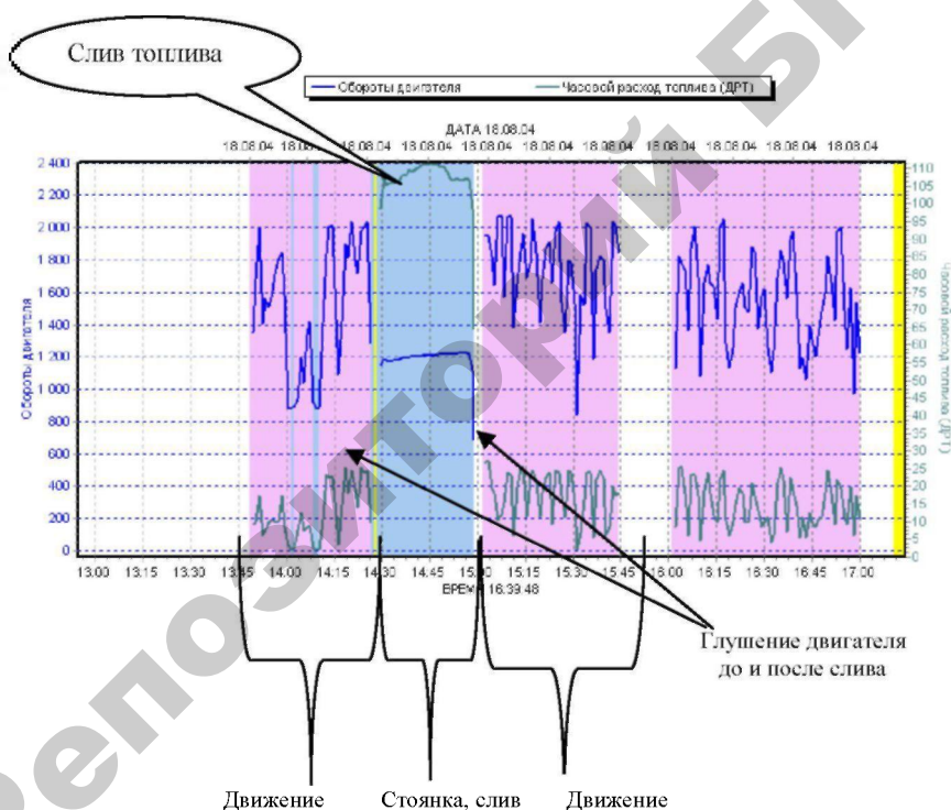
Рис. 2.65. Слив на остановленном транспортном средстве на малых оборотах. (Двигатель заведен, но между периодами нормальной работы и слива кратковременно глушился – выкручивалась пробка ТНВД. Наблюдается несоответствие оборотов двигателя и расхода топлива.)
