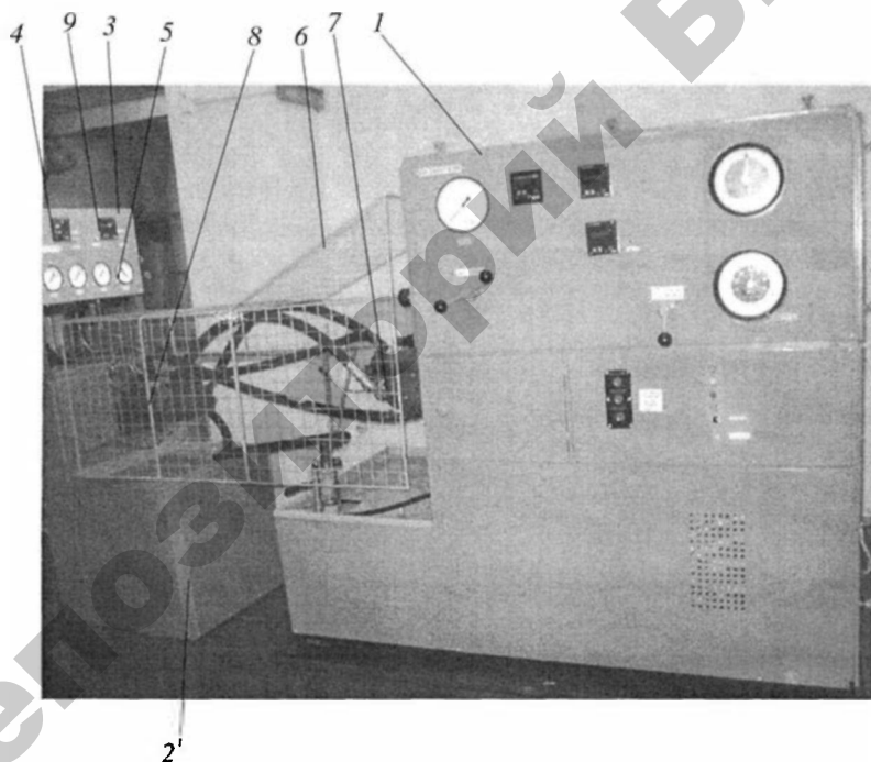
Рис. 2.1. Стенд для проверки и регулировки гидроагрегатов КИ-28097-03М: 1 – стенд; 2 – приставка к стенду; 3 – панель приборов на приставке; 4 – измеритель-регулятор ТРМ202; 5 – манометр; 6 – ограждение; 7 – гидронасос; 8 – гидромотор; 9 – измеритель ускорения
