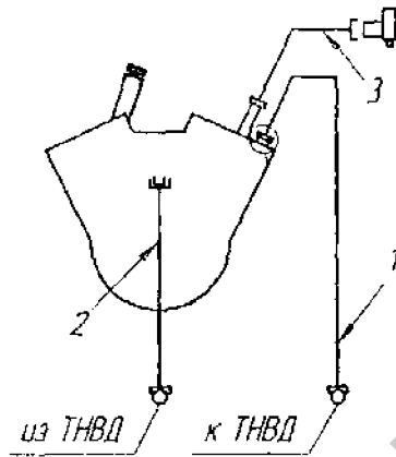
Рис. 2.17. Схема соединений топливопроводов при испытании ТНВД двигателя ЯМЗ-740 со стендовым насосом:
