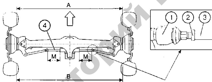
Рис. 3.65. Схема регулировки сходимости передних колес:
