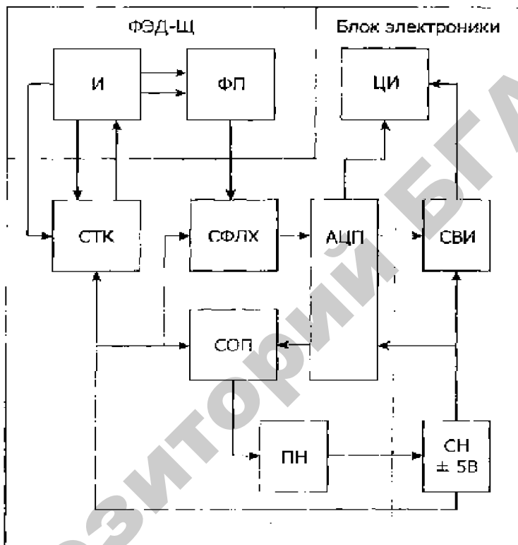
Рис. 3.78. Функциональная схема индикатора
