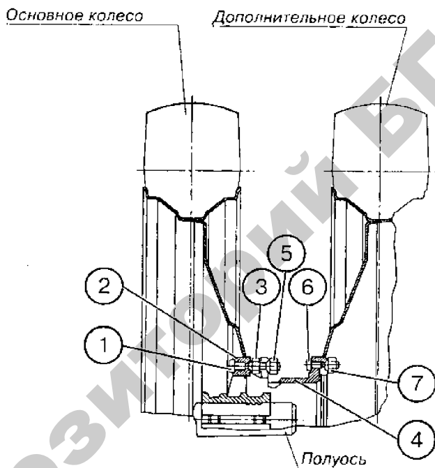
Рис. 3.62. Схема установки сдвоенных задних колес тракторов «Беларус-1522,-1523»:
