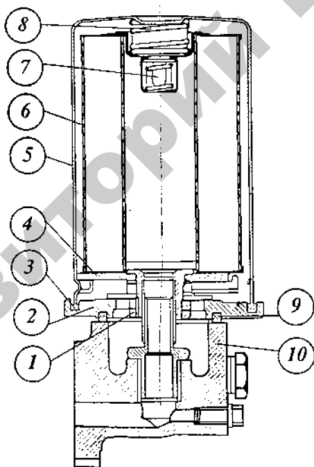
Рис. 3.14. Замена бумажного фильтрующего элемента масляного фильтра дизеля:
