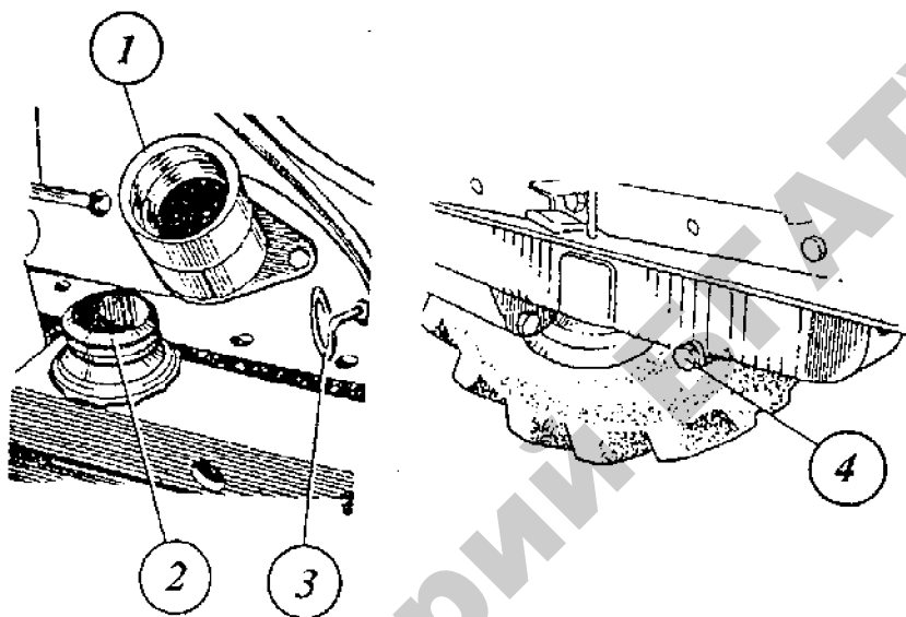
Рис. 3.12. Замена масла в картере дизеля:
