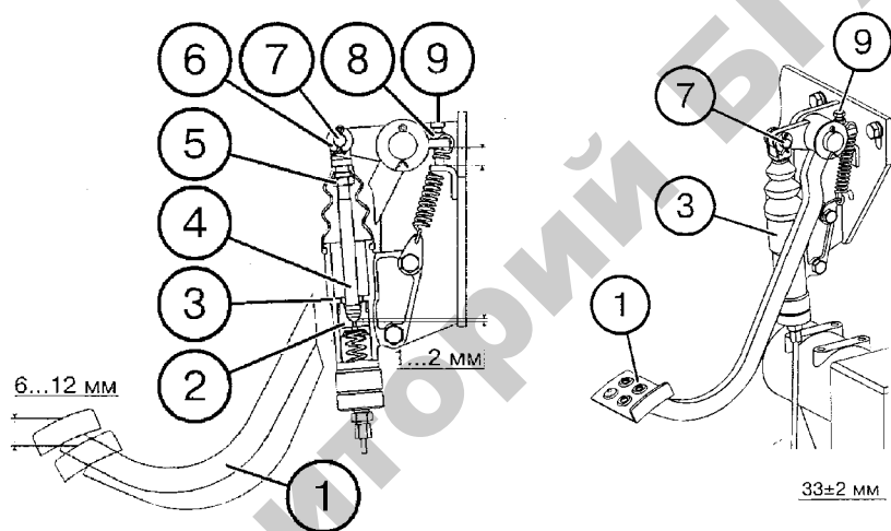
Рис. 3.40. Регулировка рабочих тормозов трактора «Беларус-1523»:
