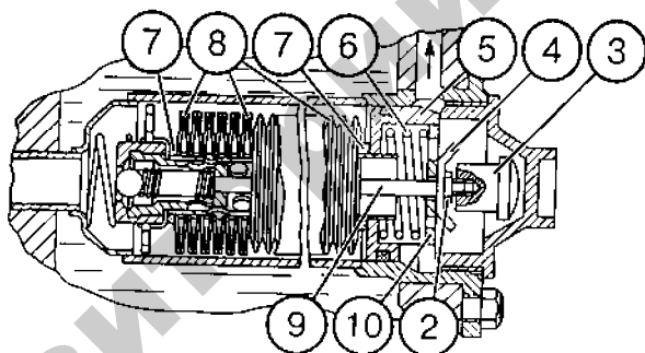
Рис. 3.21. Схема очистки сетчатого масляного фильтра КПП трактора «Беларус-1221»:
