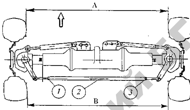
Рис. 3.27. Схема проверки сходимости передних колес трактора «Беларус-1221»:
