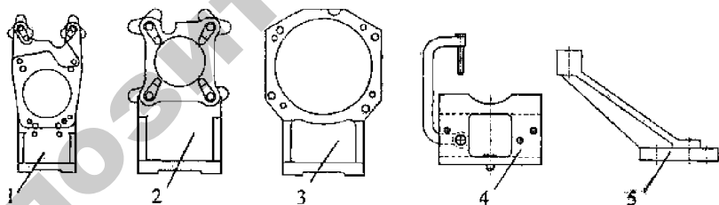
Рис. 2.14. Кронштейны для крепления топливных насосов:
