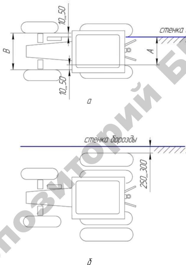
Рис. 3.66. Схема расстановки колес для агрегатирования с 5-, 7-корпусными плугами:
