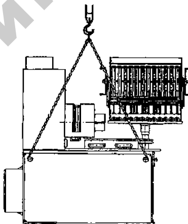
Рис. 2.13. Схема строповки
