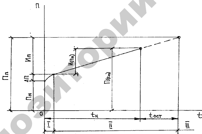
Рис. 5.1. Схема прогнозирования остаточного ресурса при известной наработке от начала эксплуатации:
