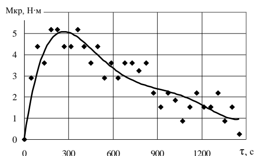
Рисунок 2 - Влияние продолжительности замеса на смену крутящего момента, при n = 0,8 \text{ с}^{-1}
