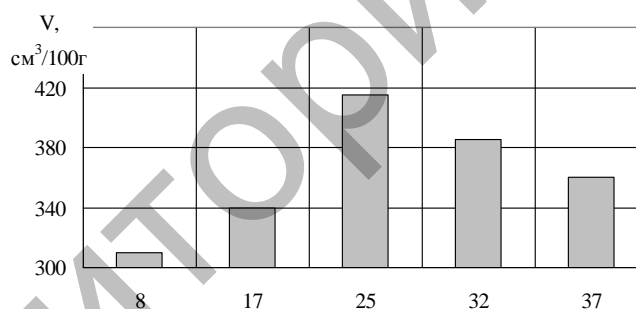
Рисунок 3 - Суммарное выделение диоксида углерода за 3 часа. брожения теста при различной удельной работе Ауд, Дж/г.
