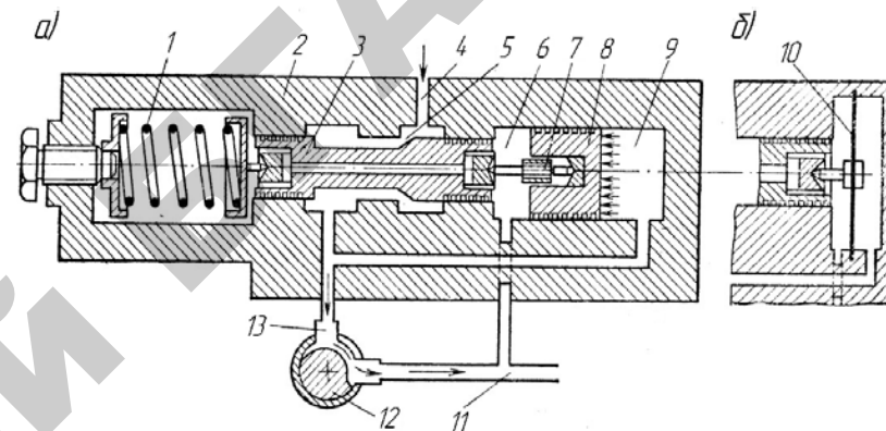
Рис. 1.3. Регуляторы потока:
