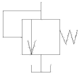
Клапан предохранительный прямого действия с нерегулируемой пружиной возврата
