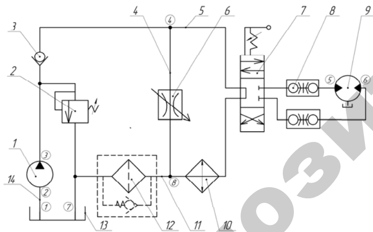
Рис. 1.5. Гидропривод с разомкнутой схемой циркуляции жидкости:
