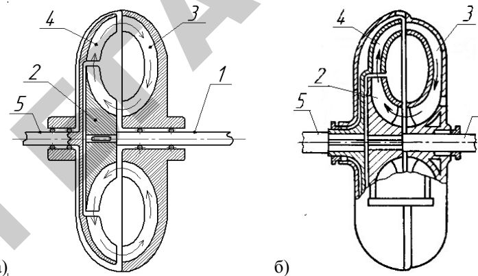
Рис. 8.3. Гидротрансформатор:
