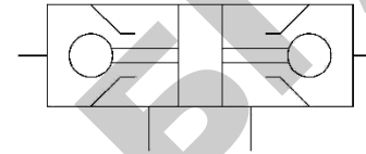
Клапан обратный управляемый двухсторонний (гидрозамок)
