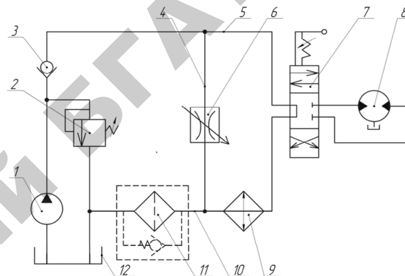
Рис. 1.1. Гидропривод с разомкнутой схемой циркуляции жидкости:
