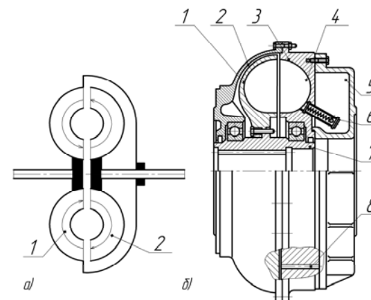
Рис. 8.1. Гидромуфта:
