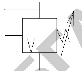
Клапан предохранительный прямого действия с регулируемой пружиной возврата
