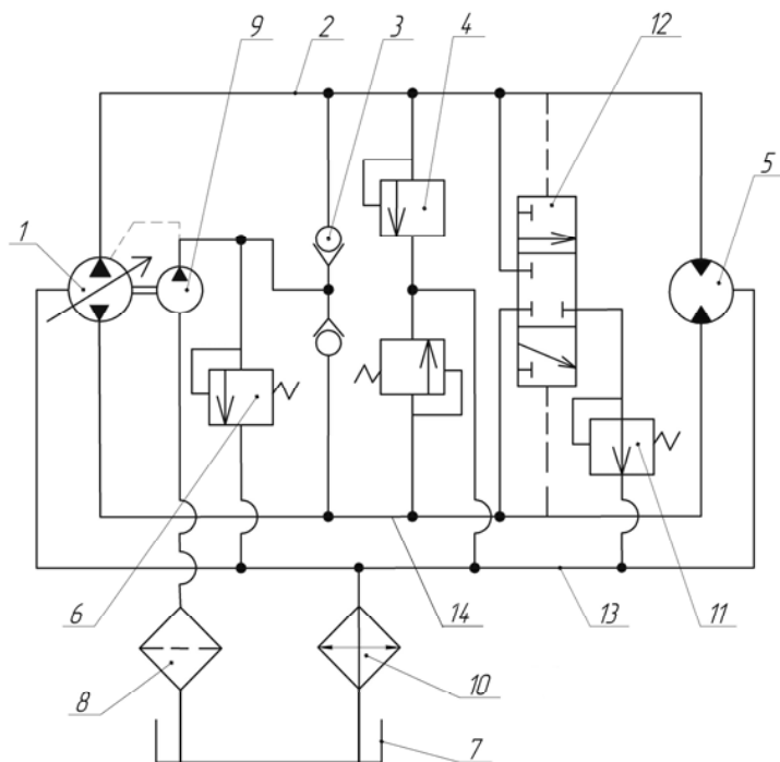
Рис. 1.2. Гидропривод с замкнутой схемой циркуляции жидкости:
