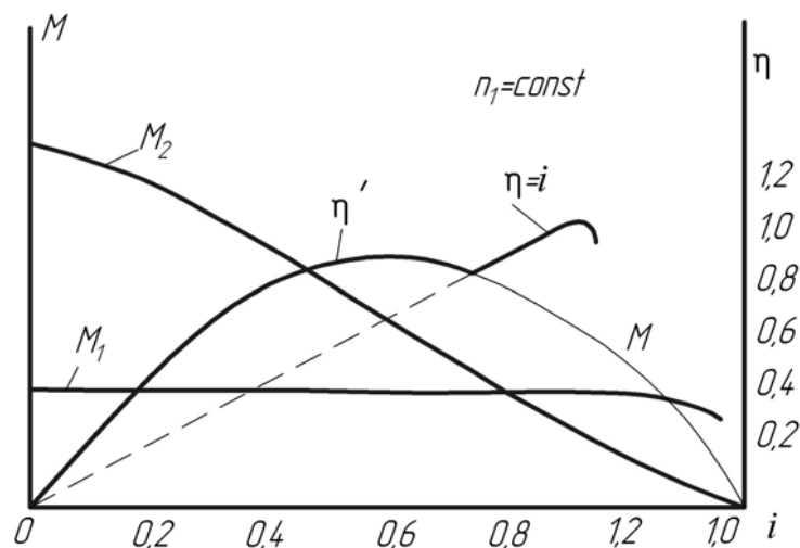
Рис. 8.5. Характеристика гидродинамической передачи
