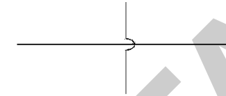
Перекрещивание трубопроводов (без соединения)
