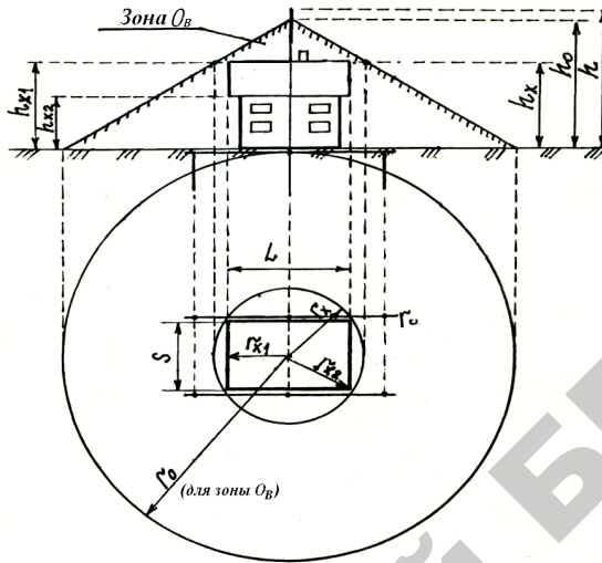
Рис. 13.6. Зоны защиты одиночного стержневого молниеотвода на сельскохозяйственном объекте
