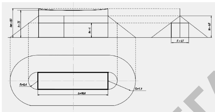
Рис. 13.10. Схема зоны защиты одиночного тросового молниеотвода
