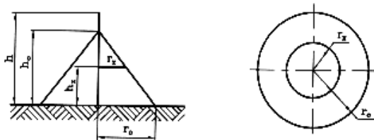
Рис. 13.1. Зона защиты одиночного стержневого молниеотвода
