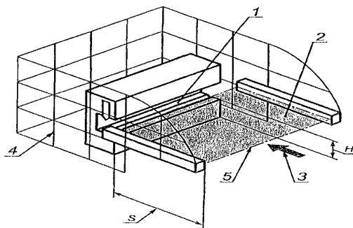
Рис. Схема параллельного приближения к зоне обнаружения: H – высота зоны обнаружения над базовой плоскостью; S – минимальное расстояние; 1 – опасная зона; 2 – зона обнаружения; 3 – направление приближения; 4 – неподвижное защитное ограждение; 5 – начало зоны обнаружения
