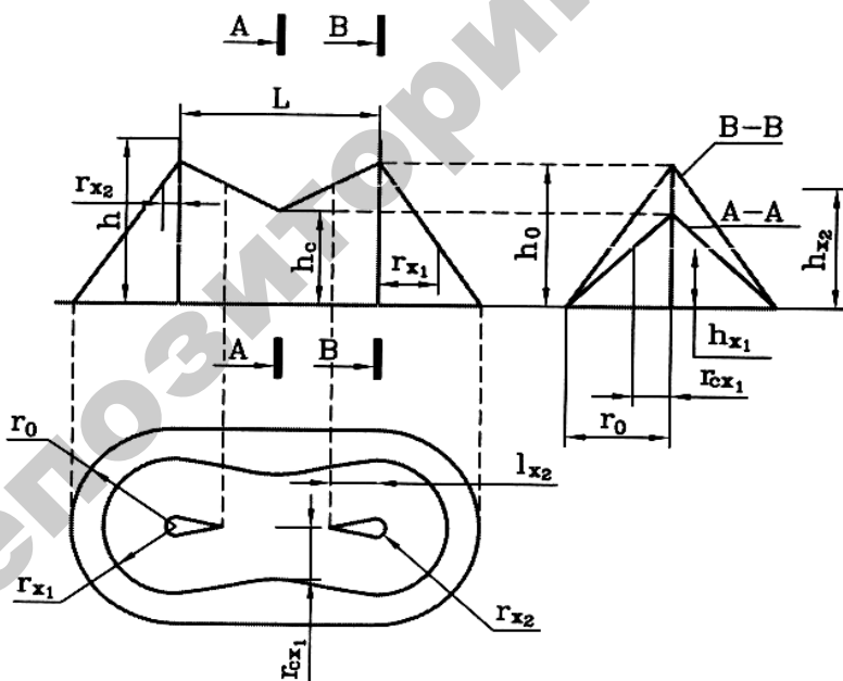
Рис. 13.4. Зона защиты двойного стержневого молниеотвода
