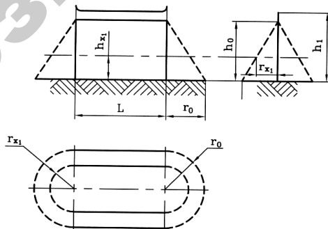
Рис. 13.3. Зона защиты одиночного тросового молниеотвода
