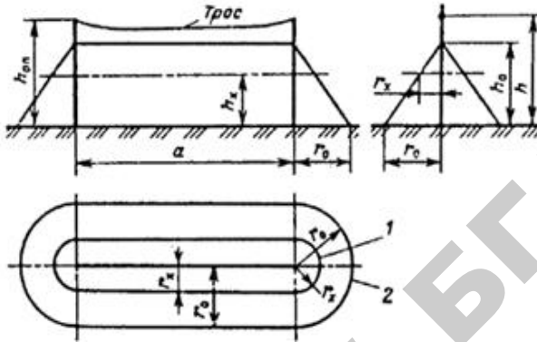
Рис. 13.8. Зона защиты одиночного тросового молниеотвода: зона 1 – граница зоны защиты на уровне h_x ; зона 2 – граница зоны защиты на уровне земли
