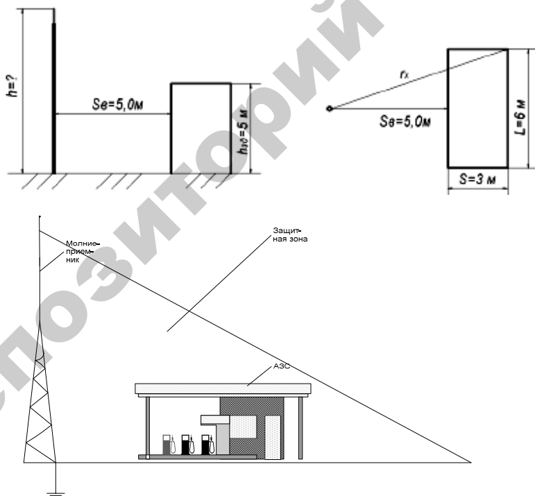
Рис. 13.9. Схема расположения молниеотвода
