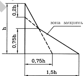
Рис. 13.2. Построение зоны защиты стержневого молниеотвода упрощенным методом
