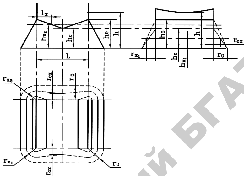
Рис. 13.5. Зона защиты двойного тросового молниеотвода
