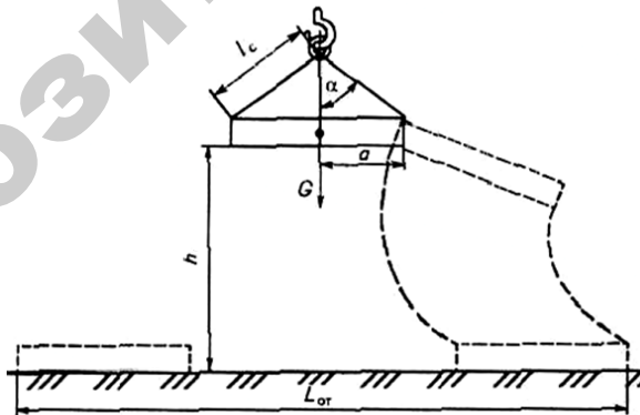
Рис. Схема определения границ опасной зоны при обрыве стропа грузоподъемной машины ( G – сила тяжести)
