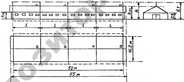
Рис. 13.7. Молниезащита коровника
