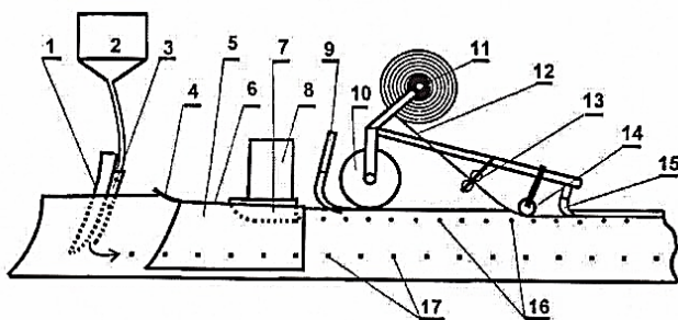
Рисунок 1 – Схема сеялки
