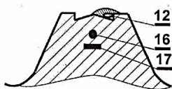
Рисунок 4 – Схема гребня с расположением поливного шланга, семян и удобрения
