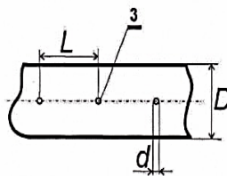
Рисунок 6 – Расположение водовыпусков
