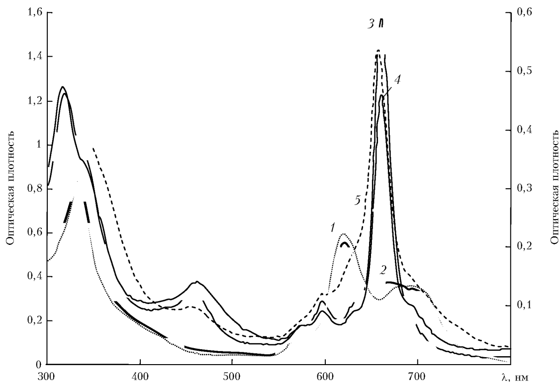
Рис. 4. Спектры поглощения \text{LuPc}_2 в ДМСО: до облучения – 1, после облучения ХеСІ-лазером – 2; в хлороформе: до облучения – 3, после облучения ХеСІ-лазером – 4; в этаноле + 0,2% НСІ без облучения – 5; 1, 2 – правая шкала, 3–5 – левая шкала
