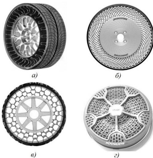
а) – MichelinTweel; б) – BridgestoneAirFree; в) – PolarisResilientTechnologies; г) – HankookI-Flex
