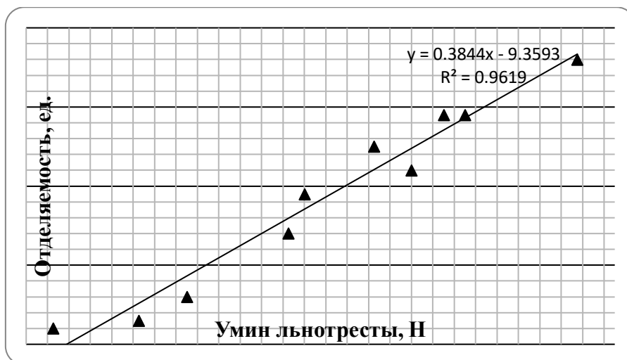
Рис. 1. Аппроксимация зависимости отделимости льнотресты от умина.
