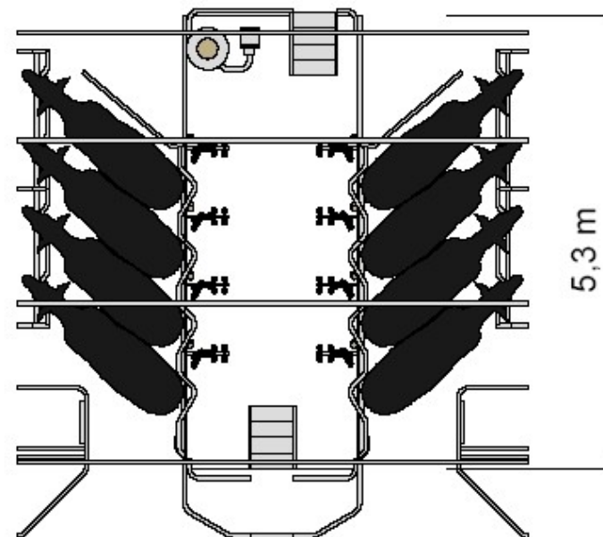
Рис. 1.20. Доильный зал типа «Ёлочка»
