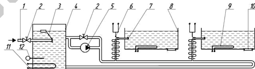
Рис. 1.16. Схема циркуляционного водопровода с подогревом воды и «уровневыми поилками»:
