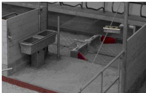
Рис. 1.15. Опрокидывающаяся поилка «Farmtec» с подогревом
