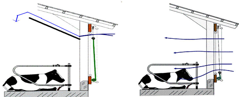
Рис. 1.8. Регулирование объема поступающего воздуха с помощью специальных штор
