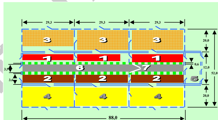
Рис. 1.34. Схема реконструированного помещения для содержания коров с телятами и телят послеотъемного периода (полезная площадь для коров с телятами – 321 м 2 на 40–50 коров с телятами; полезная площадь для телят послеотъемного возраста – 321 м 2 на 70 гол.):
