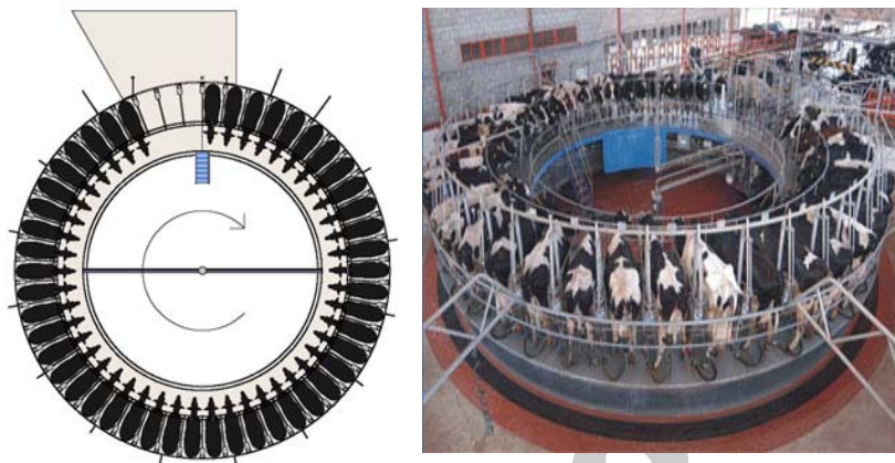
Рис. 1.23. Доильный зал типа «Карусель»–«Бок в бок»
