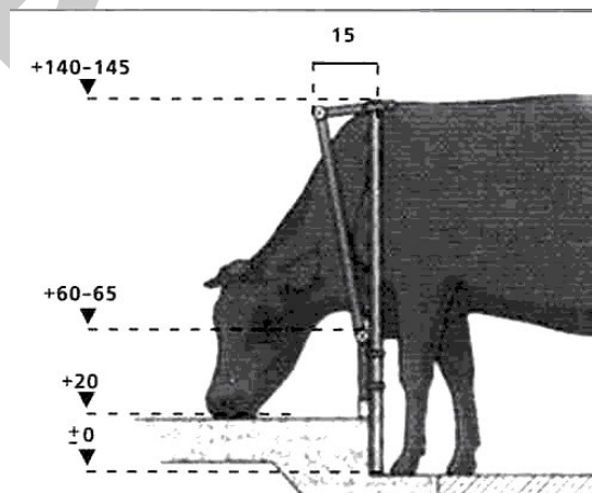
Рис. 1.14. Фиксирующее ограждение и параметры его расположения
