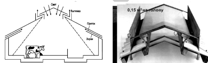
Рис. 1.9. Светоаэрационный конек с ветрозащитными щитками
