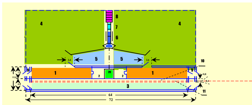
Рис. 1.33. Схема реконструированного помещения для мясного скота под родильное отделение:
