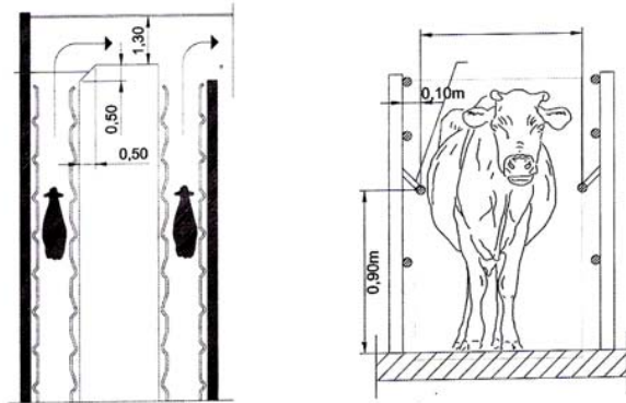
Рис. 1.27. Поворотный коридор из доильного зала и его параметры
