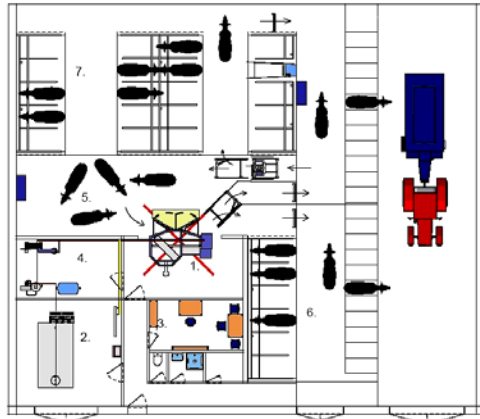
Рис. 1.26. Планировка коровника с совмещенным доильным залом, оборудованным «роботом-дойаром»
