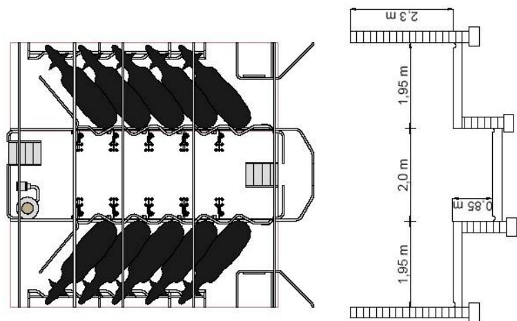
Рис. 1.19. Доильный зал типа «Ёлочка»
