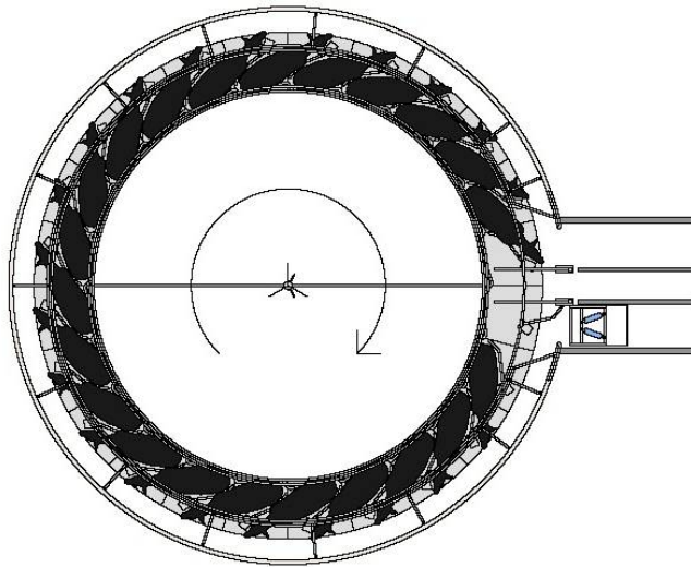
Рис. 1.22. Доильный зал типа «Карусель»–«Елочка»
