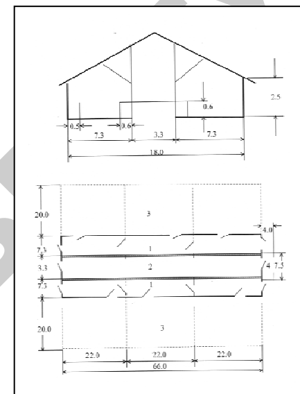
Рис. 1.32. Схема здания из облегченных конструкций:
