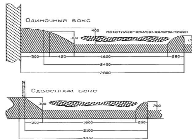
Рис. 1.11. Конструкция пола боксов
