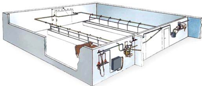
Рис. 1.17. Линейный молокопровод в коровнике с привязным содержанием
