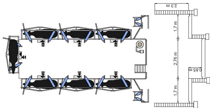
Рис. 1.18. Доильный зал типа «Автотандем»
