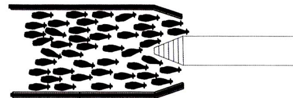
Рис. 1.24. Разделение входа из зала ожидания на доильные места
