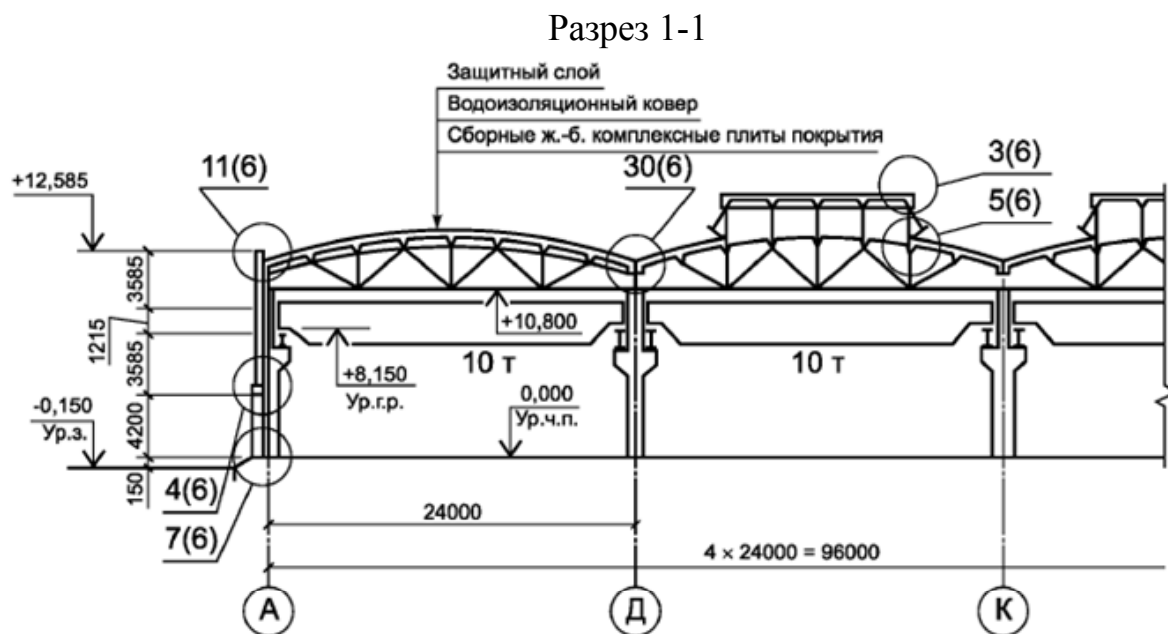
Рисунок У.1 – Пример выполнения разреза одноэтажного производственного здания
