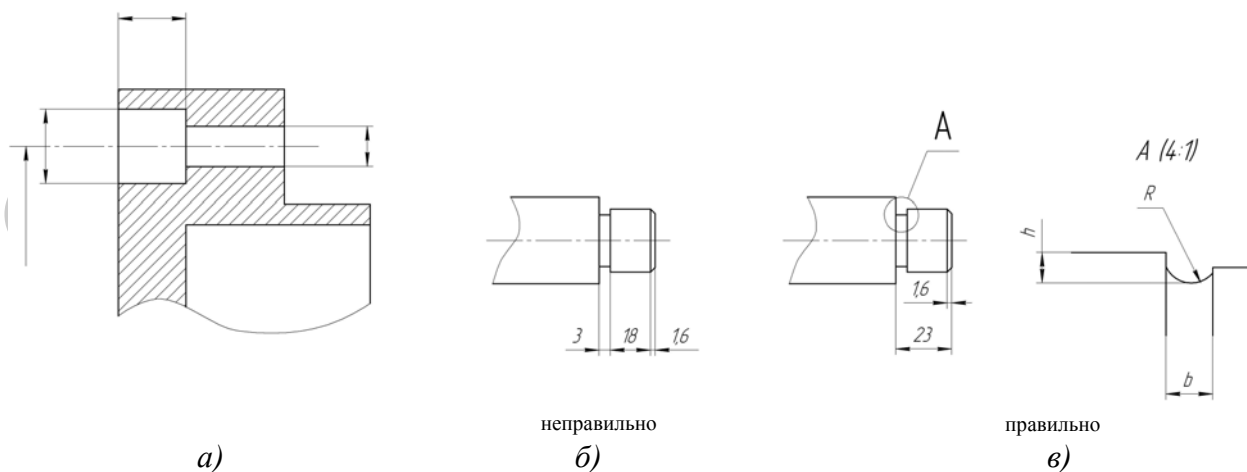
Рисунок 6.6 – Примеры нанесения размеров на чертежах
