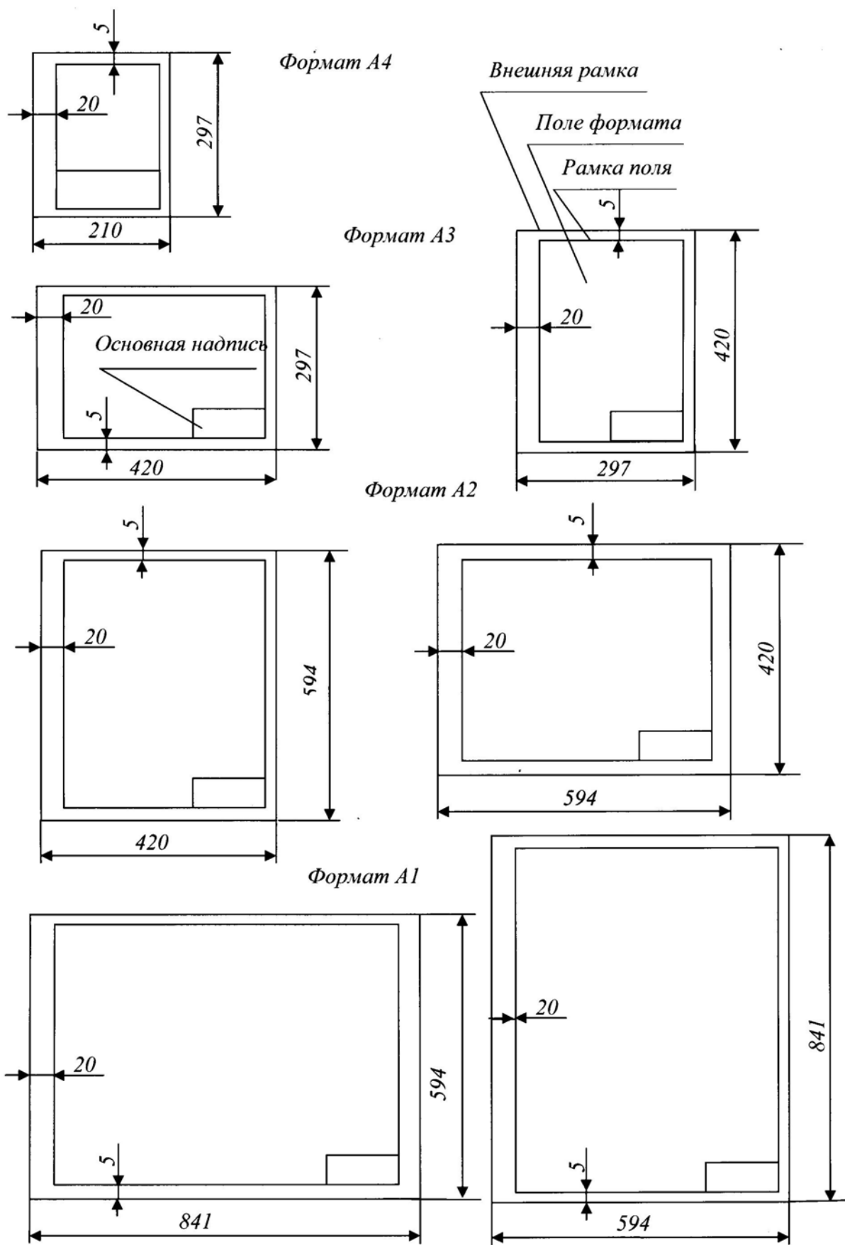
Рисунок 6.1 – Форматы листов
