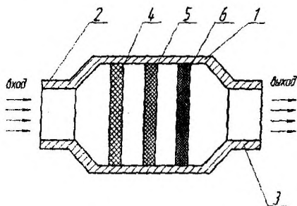
Рис. 1. Схема искрогасителя:
