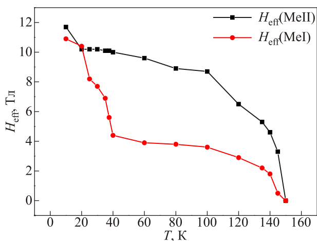
Рис. 2. Зависимость величин эффективных магнитных полей на ядрах атомов железа в октаэдрических (FeI) и тригонально-бипирамидальных (FeII) позициях от температуры.
