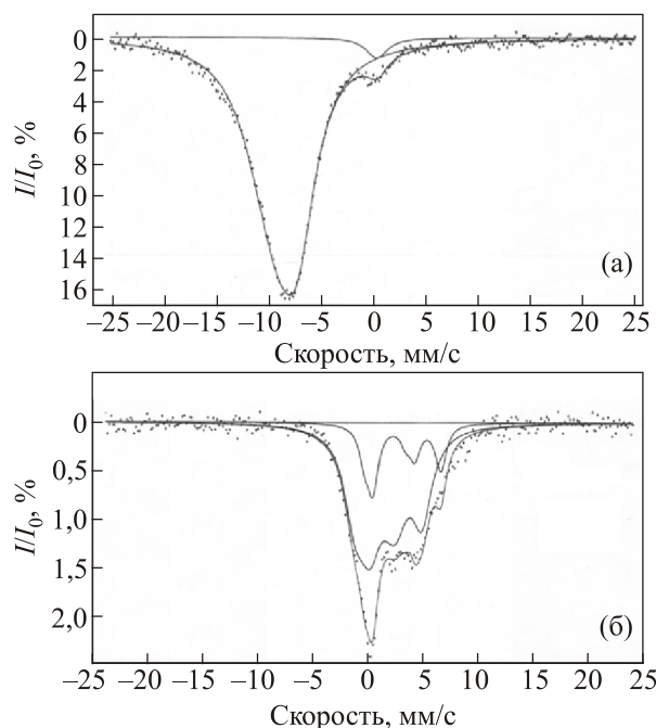
Рис. 3. Мессбауэровские спектры антимонида железа на изотопах ^{121}\text{Sb} (a) и ^{119}\text{Sn} (б) при T = 77\text{ K} .
