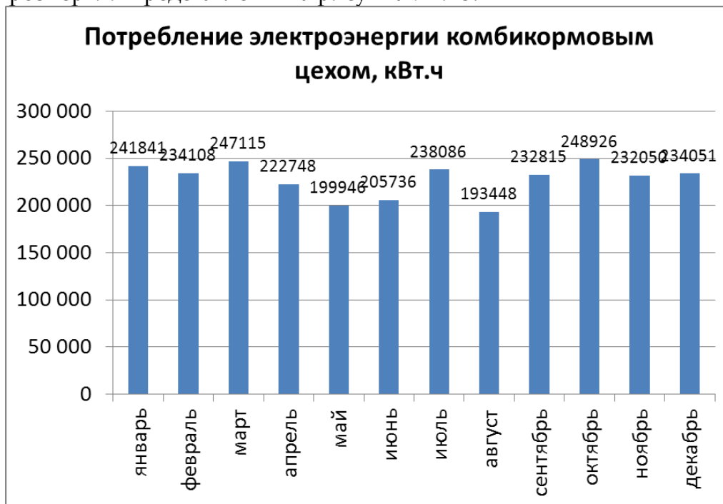
Рис. 2 Годовое потребления электроэнергии комбикормовым цехом
