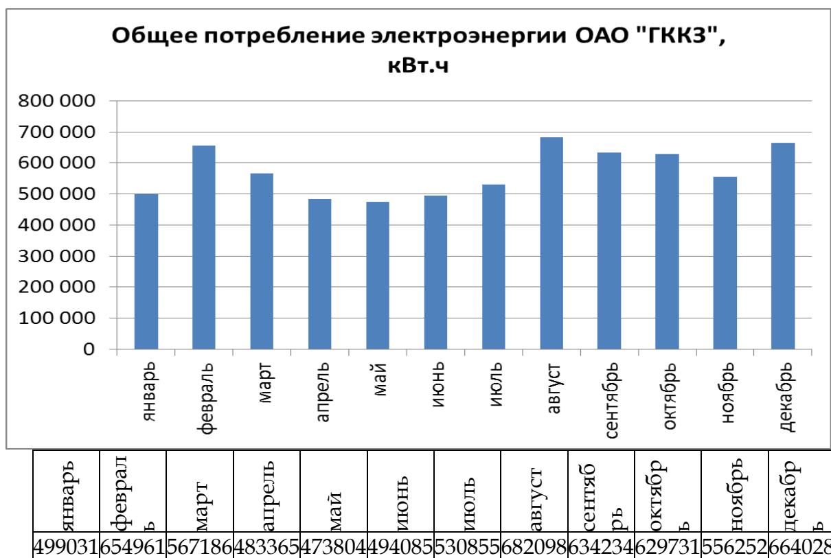
Рис. 1 Годовое потребления электроэнергии ОАО «Глубокский комбикормовый завод»
