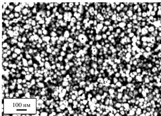
Рис. 1.2. Поверхность тонкого нанокристаллического покрытия оксида циркония ( ZrO_2 ), сформированного золь-гель методом. Микроизображение получено методом просвечивающей электронной микроскопии
