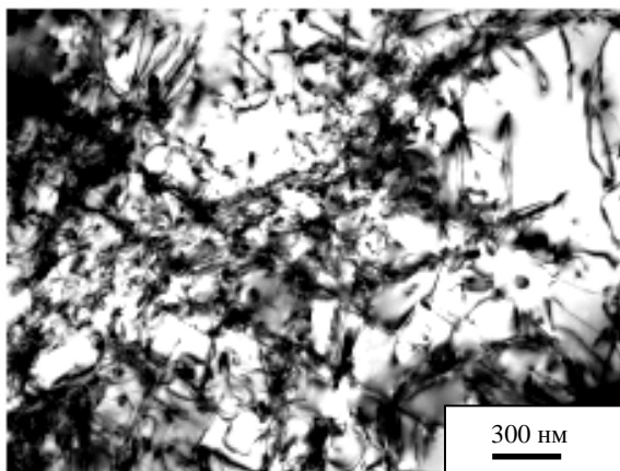
Рис. 1.3. Структура пера турбинной лопатки из жаропрочного никелевого сплава СС-70. Микроизображение получено методом просвечивающей электронной микроскопии
