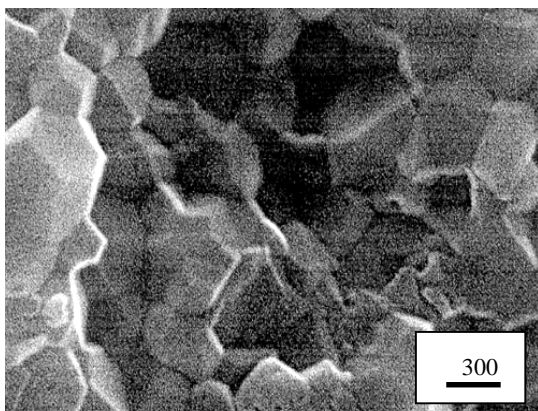
Рис. 1.7. Микроструктура излома нанокристаллической керамики на основе оксида алюминия Al_2O_3 , полученной прессованием и последующим спеканием нанопорошков. Микроизображение получено с помощью сканирующего электронного микроскопа
