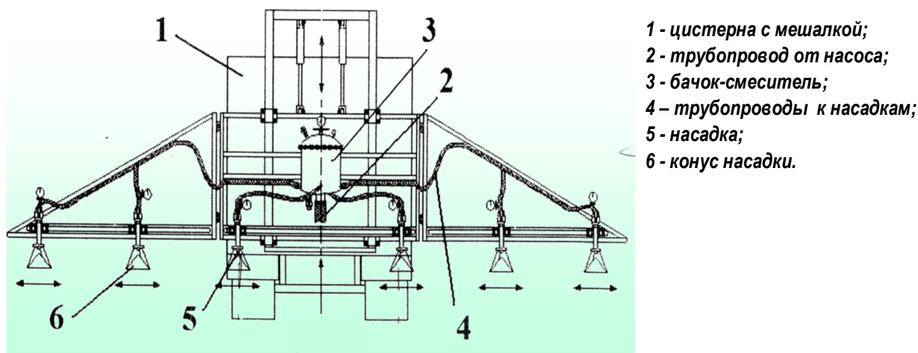
Рисунок 4 – Высевальная штанга с бачком-смесителем
