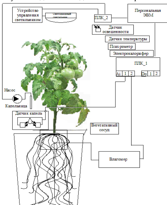
Рисунок 2 – Конструктивное исполнение экспериментальной установки.
