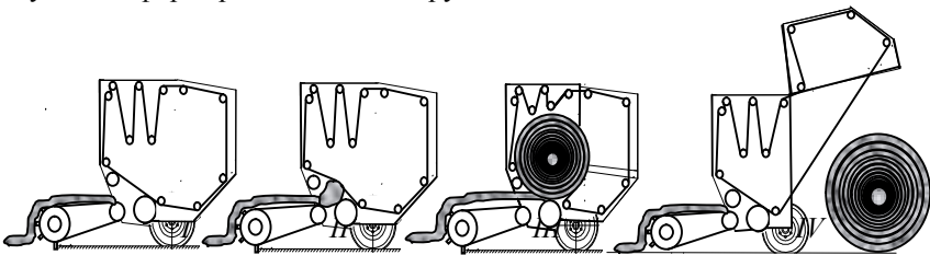
Рисунок 1 – Схема технологического процесса I – подача льносырья в пресс-камеру; II–III – формирование рулона; IV – выгрузка рулона
