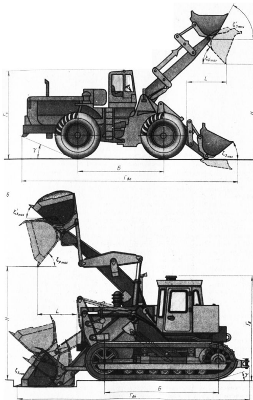
Рисунок 1 – Обозначения основных размерных технико-эксплуатационных параметров погрузчиков: а) пневмоколесных (с параллелограммным рычажным механизмом); б) гусеничных (с перекрестным рычажным механизмом)
