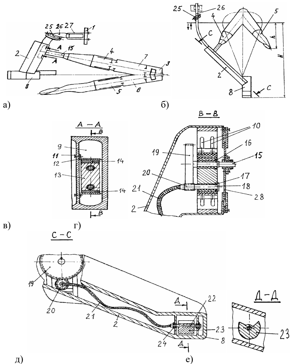
Рисунок 1 – Корнеплодоизвлекающее устройство
