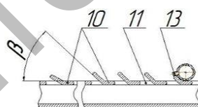
Рисунок 2 - Выгрузная горловина, местный вид I
