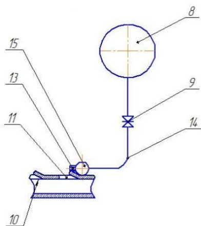
Рисунок 4 – Емкость мобильного измельчителя с дозирующим устройством, соединенная трубопроводами с соплами
