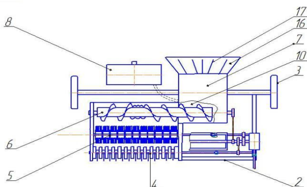
Рисунок 3 – Модернизированный измельчитель, вид сверху
