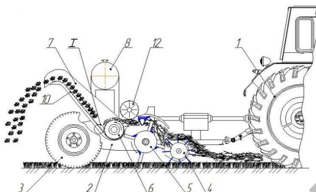
Рисунок 1 - Технологическая схема модернизированного измельчителя
