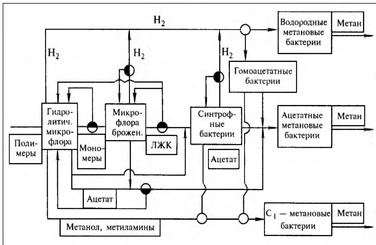
Рисунок 23 – Схема действия микробного сообщества при получении биогаза (по Ю.А. Горбунову)
