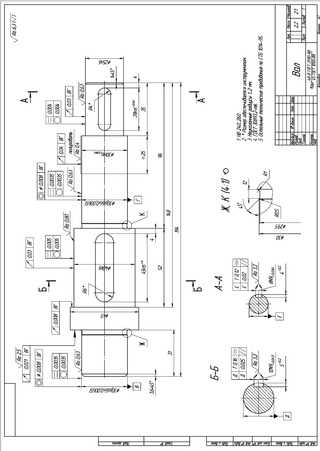
Рисунок 1.22 – Пример выполнения чертёжа вала
