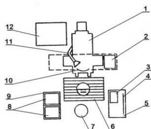
Рисунок Ю.2 – Планировка рабочего места сверловщика
