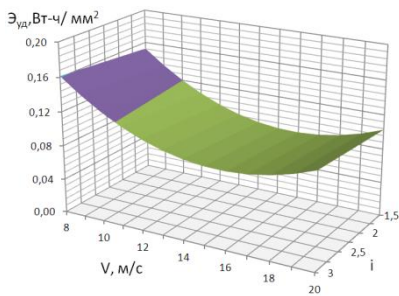
Рисунок 2 – Зависимость удельной энергоёмкости от скорости быстро вращающегося вальца V_{\delta} и отношения окружных скоростей вальцов i при межвальцовом зазоре 0,4 \text{ мм}
