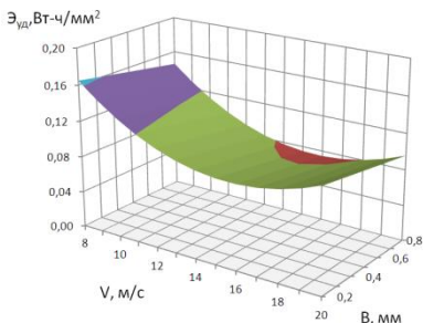
Рисунок 1 – Зависимость удельной энергоёмкости от окружной скорости быстро вращающегося вальца V_{\delta} и межвальцового зазора B при отношении окружных скоростей вальцов i = 2
