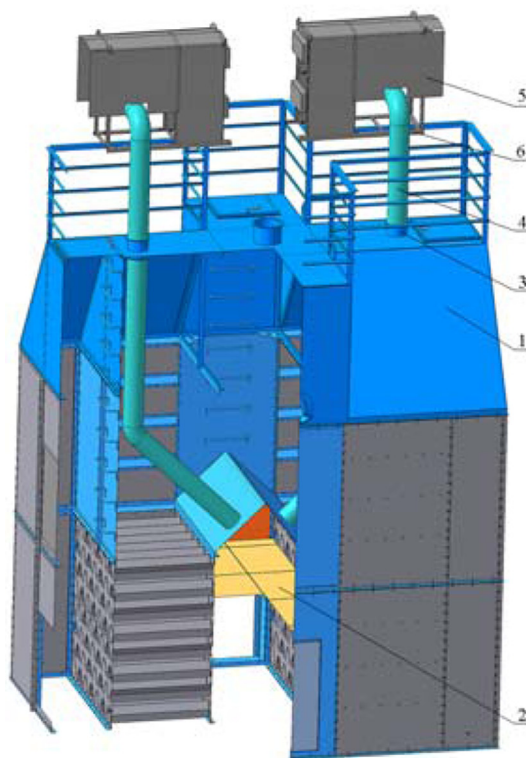
Рис. 6. Сушилка с использованием озонородушной смеси
