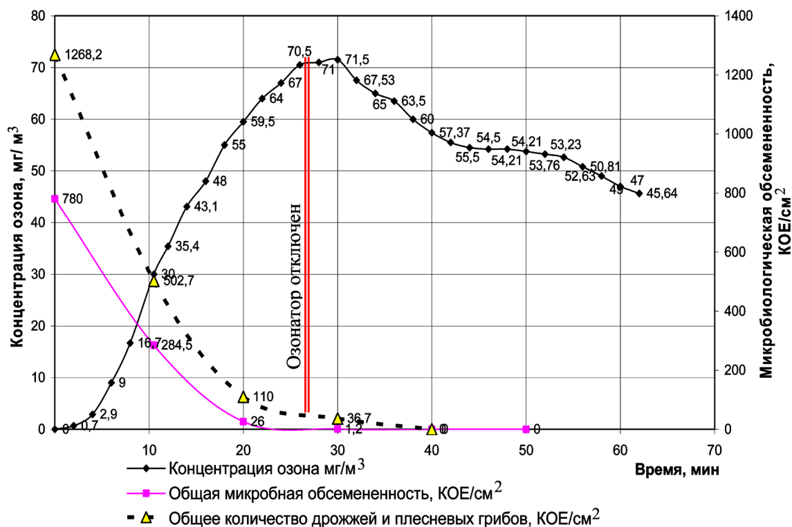
Рис. 5. Зависимость микробиологической обсемененности приточной емкости на УП «Можейково» объемом 12 м³ от концентрации и времени его воздействия
