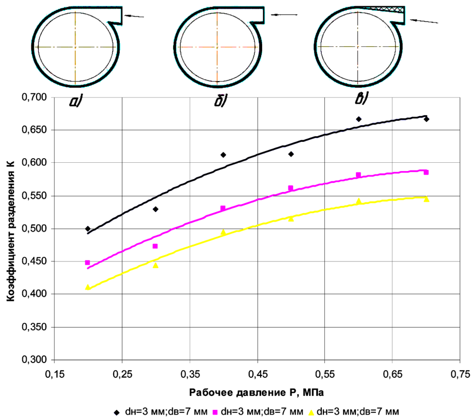
Рис. 3. Зависимость коэффициента разделения крахмальной суспензии от рабочего давления: a – коническое сходящееся отверстие; b – цилиндрическое отверстие; c – цилиндрическое отверстие под углом 45°
