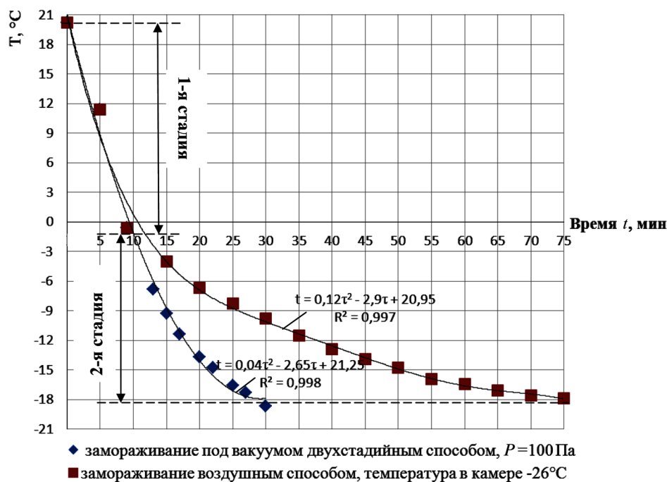
Рис. 1. Зависимости температуры в центре пельменей от продолжительности их замораживания воздушным способом и двухстадийным способом под вакуумом
