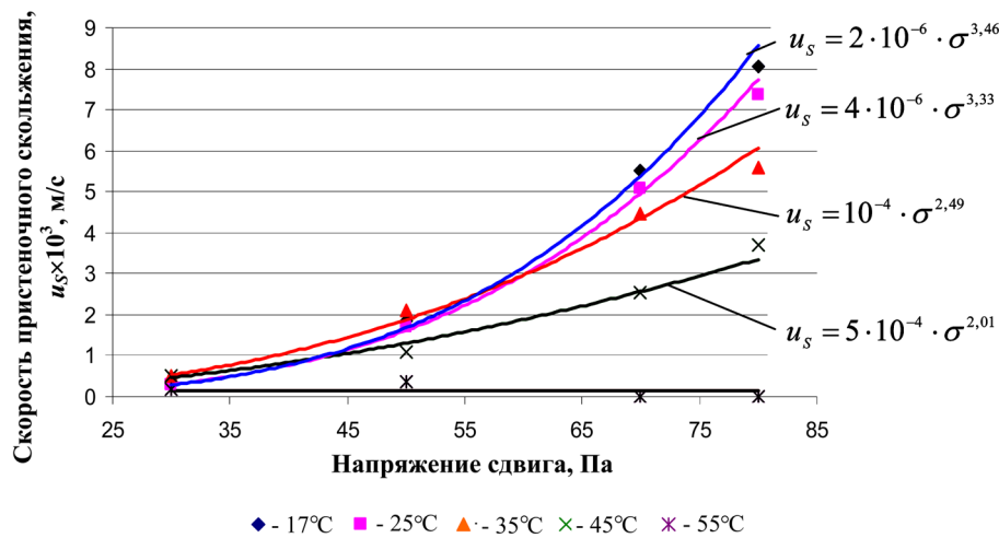
Рис. 4. Зависимость скорости жидкотекучего продукта (кетчупа) от напряжения сдвига при различных температурах
