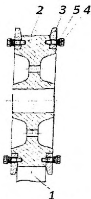
Рис. 1. Крановое колесо в разрезе
